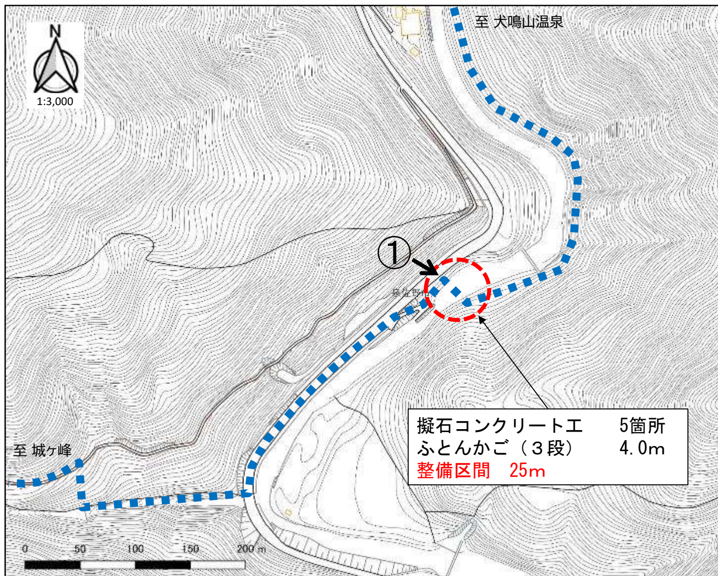
【平面図】
