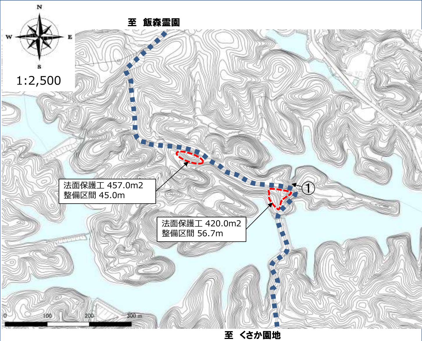
【平面図】
