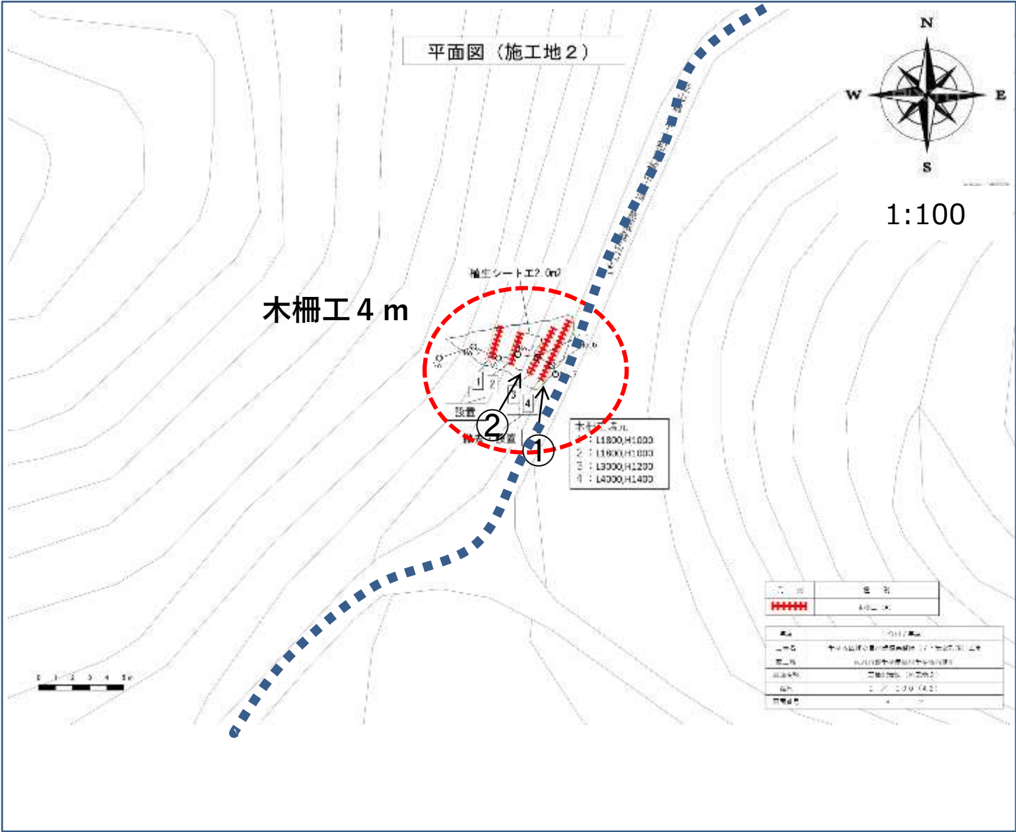
【平面図】
