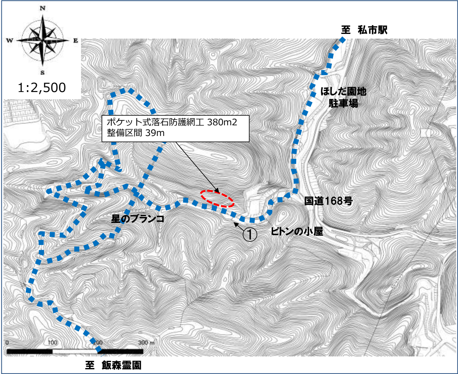
【平面図】
