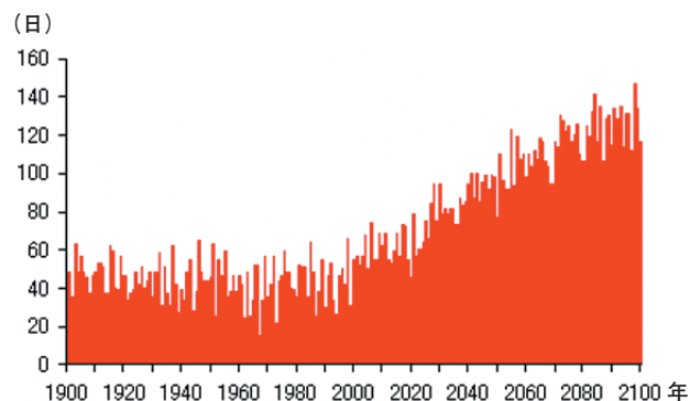
図1-16 日本の真夏日日数の変化
