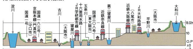
東西断面図(国道308号沿)
