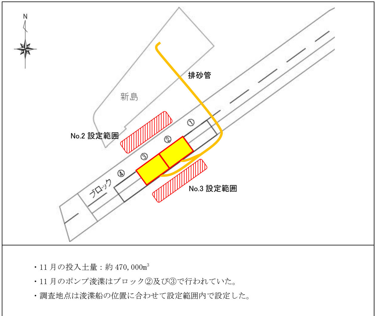
図一(3) 工事箇所及びNo. 2, No. 3の設定範囲(11月)
