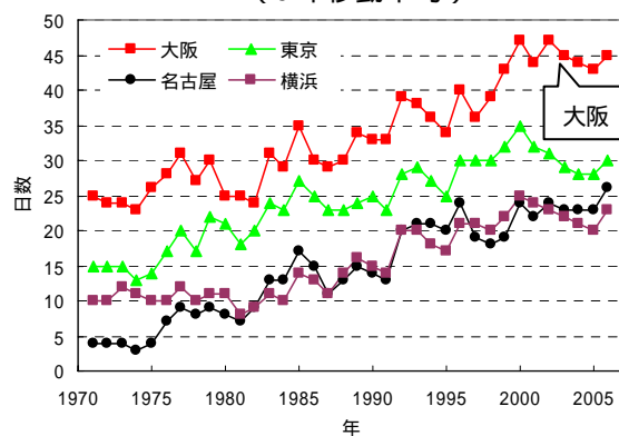
図-14 大都市における熱帯夜数 (5年移動平均)
