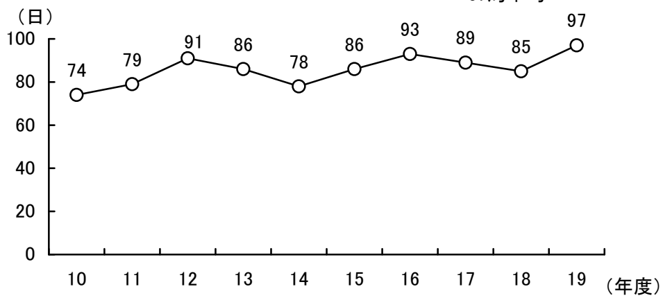
4-5 昼間の光化学オキシダント濃度が0.06ppmを超えた日数の推移
