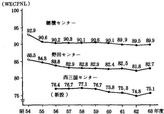
図 2-6-3 航空機騒音の常時測定結果の推移
