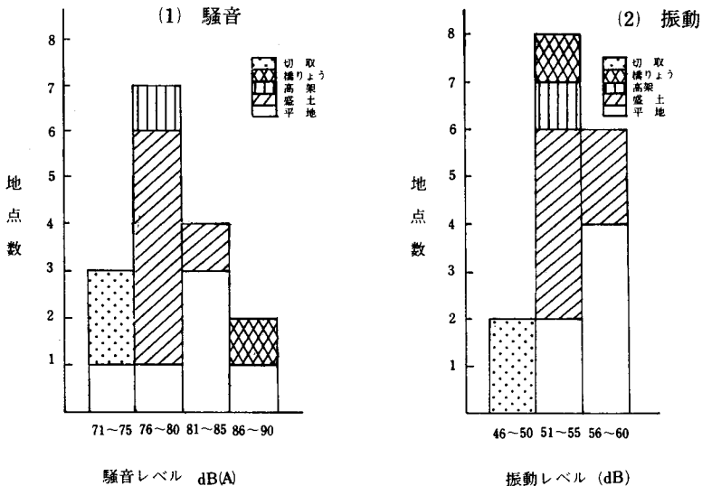
図3-4-1 鉄軌道の騒音レベル及び振動レベルの頻度分布
