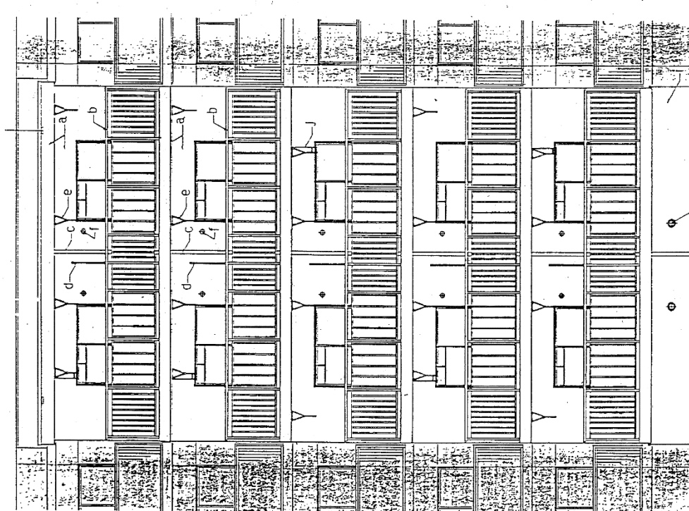
立面詳細図 1/50
