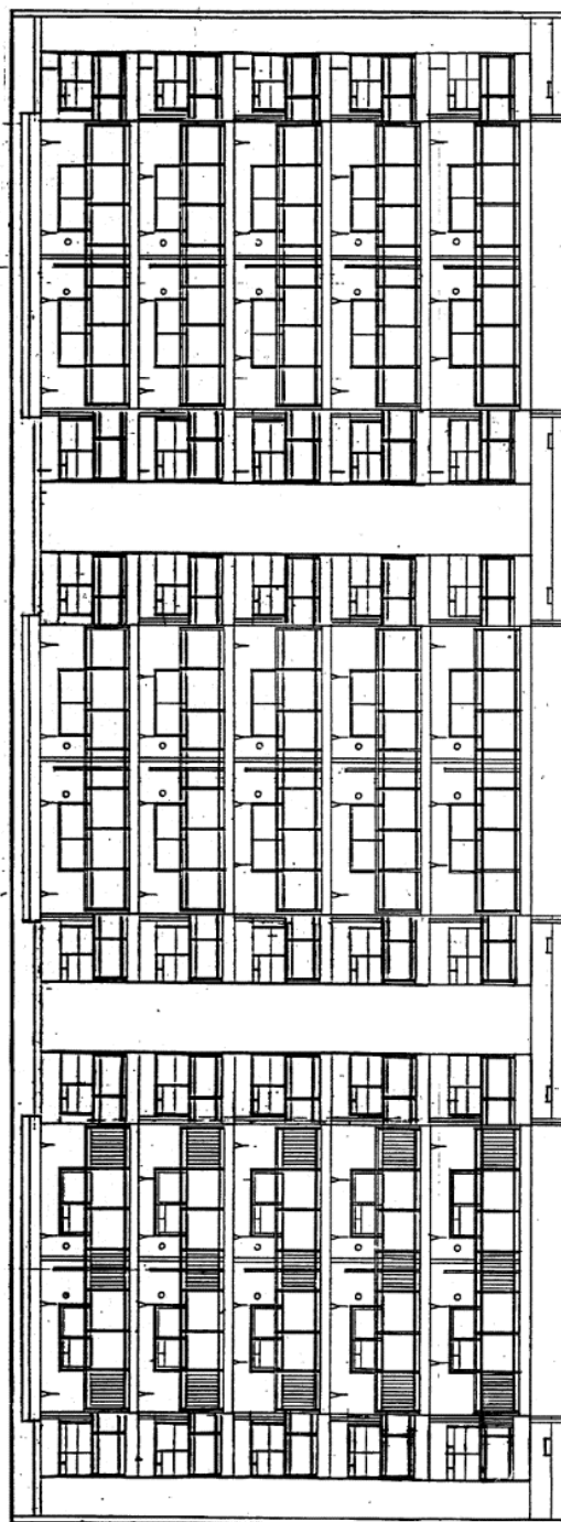
15号楼 南侧立面图 1:100
