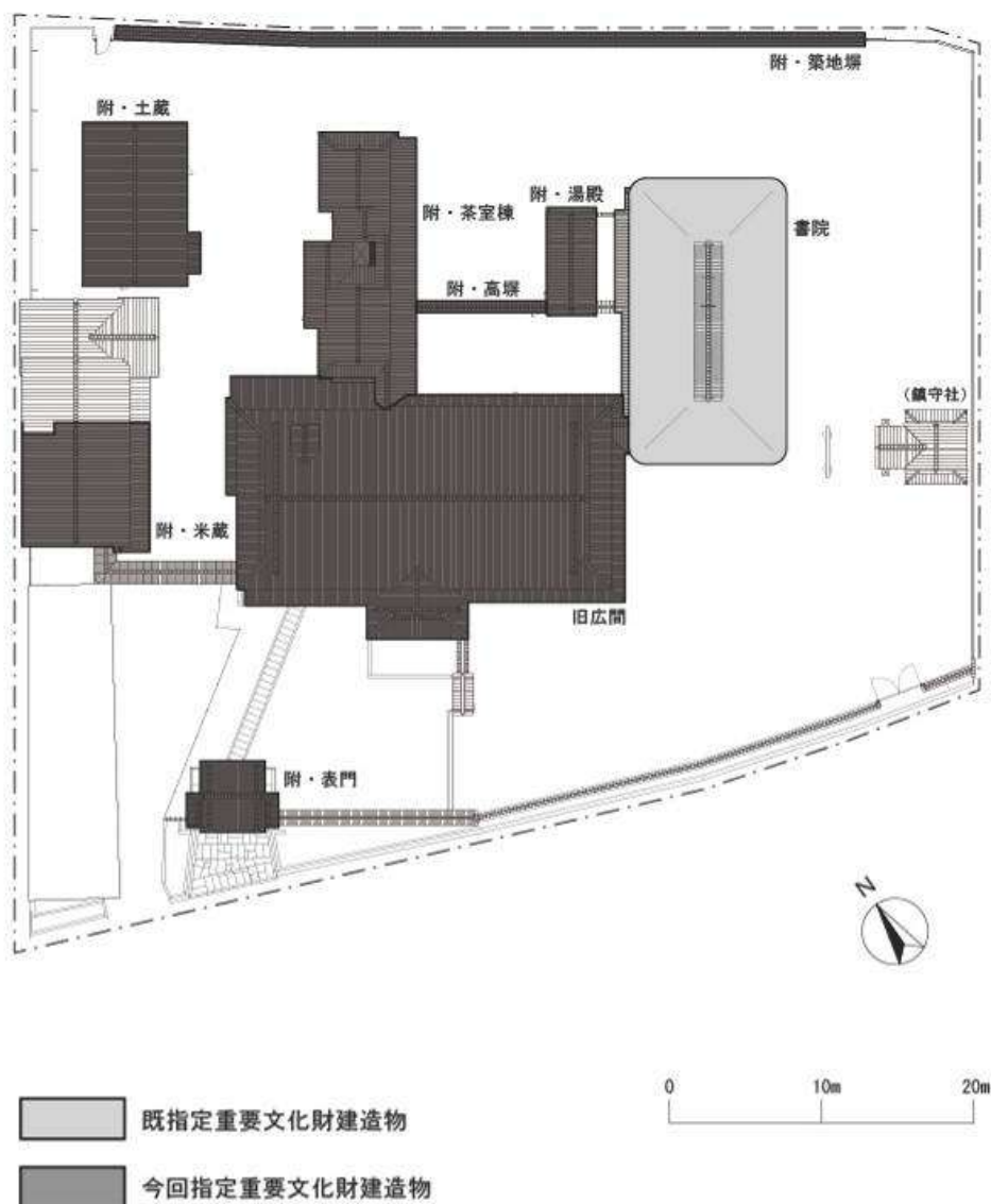
降井家住宅 建物配置図
