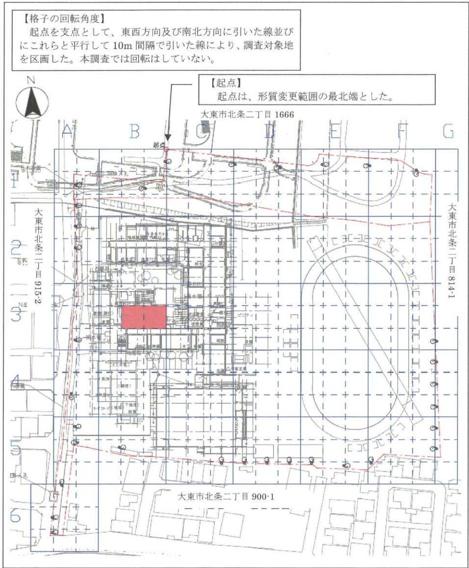
区域指定平面図 大東市北条二丁目 909 番 1 及び 912 番 1 の各一部
