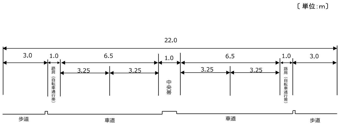
標準断面図
