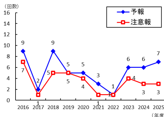
光化学スモッグの発令回数の推移
