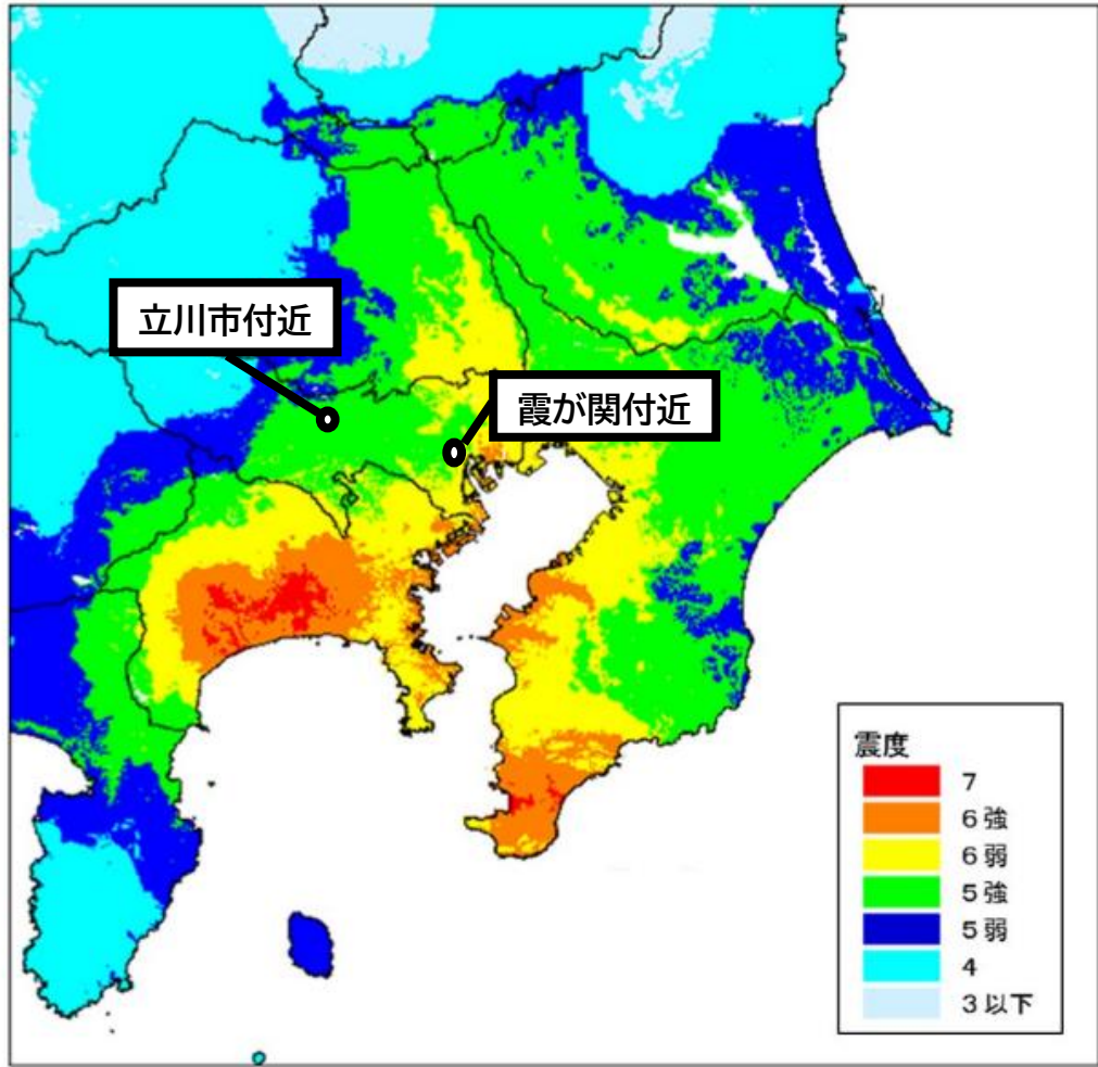
震度分布（大正関東地震）
