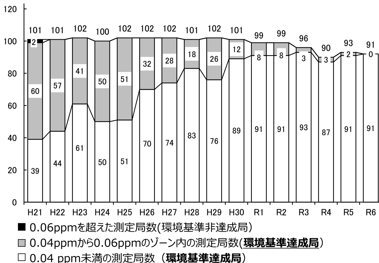
図1. 府内全局の \text{NO}_2 の環境基準達成状況の推移 (年間98%値の分布状況)
