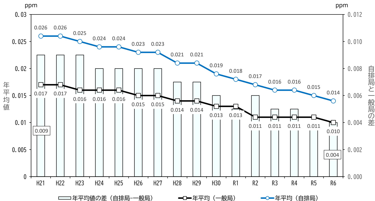
図3. \text{NO}_2 濃度（年平均値）の経年変化【大阪府全域】
