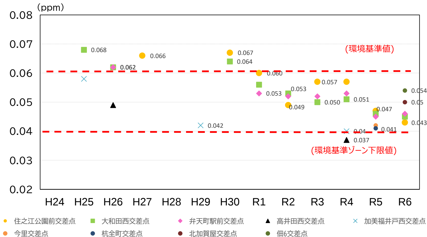
図10. NO 2 日平均値の年間98%換算値の推移
