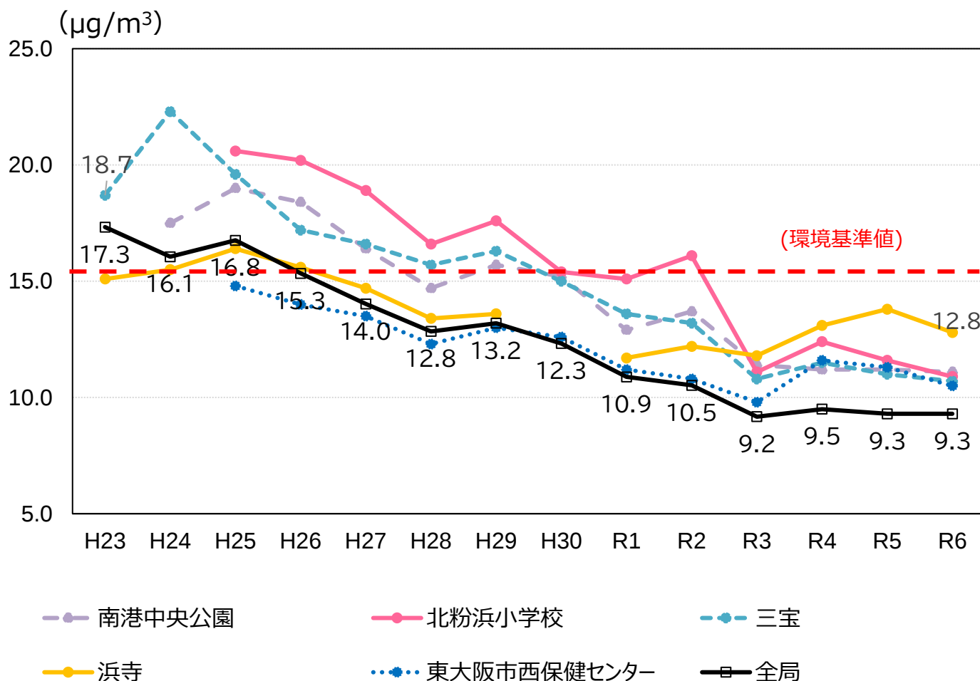
図8. PM2.5 (年平均値) の上位5局 (令和6年度) と全局平均の推移
