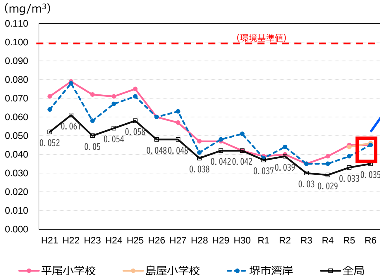
図5. SPM長期評価値 (年間2%除外値) の上位3局 (令和6年度) と全局平均の推移
