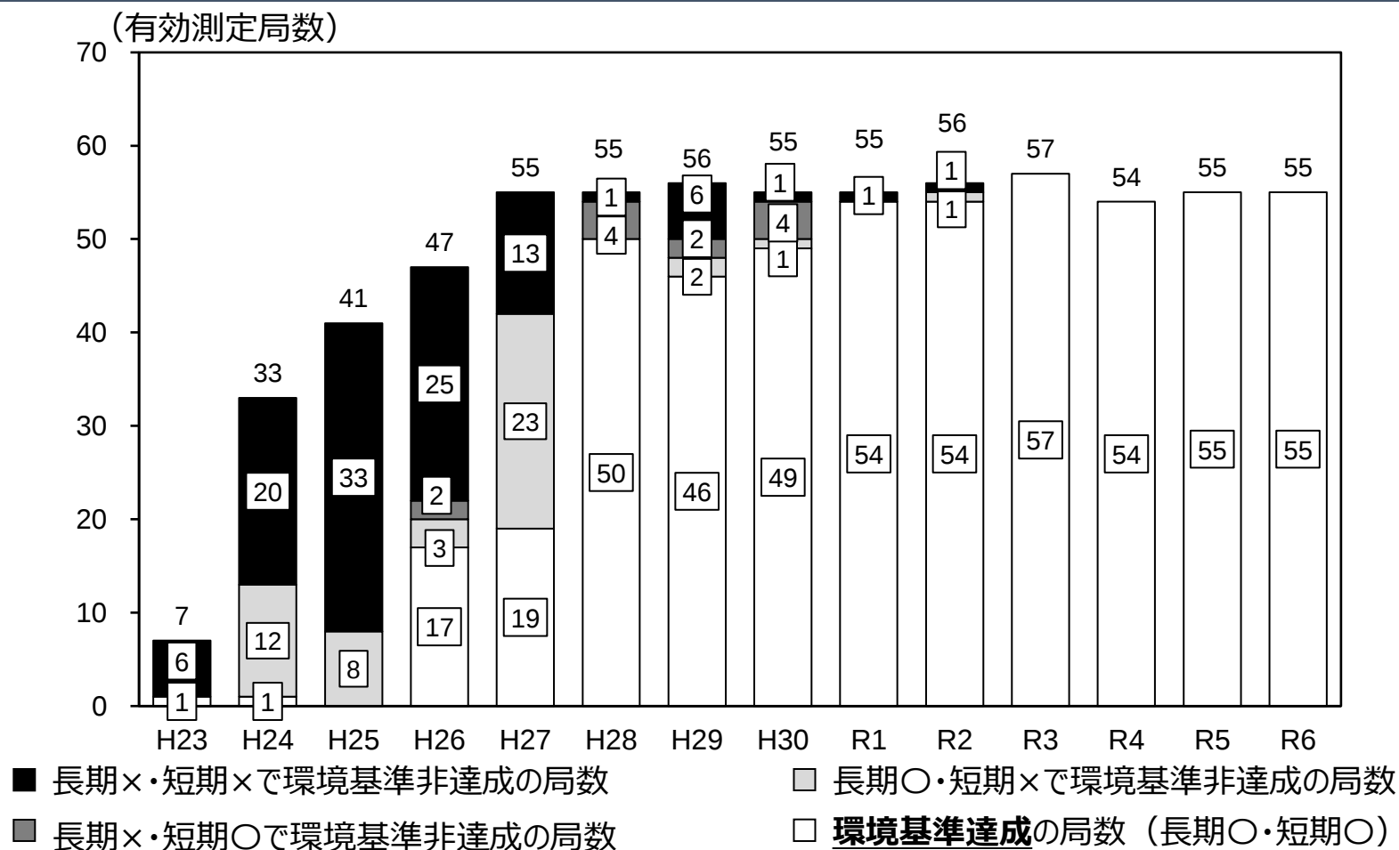
図7. 府内全局のPM2.5の環境基準達成状況の推移
