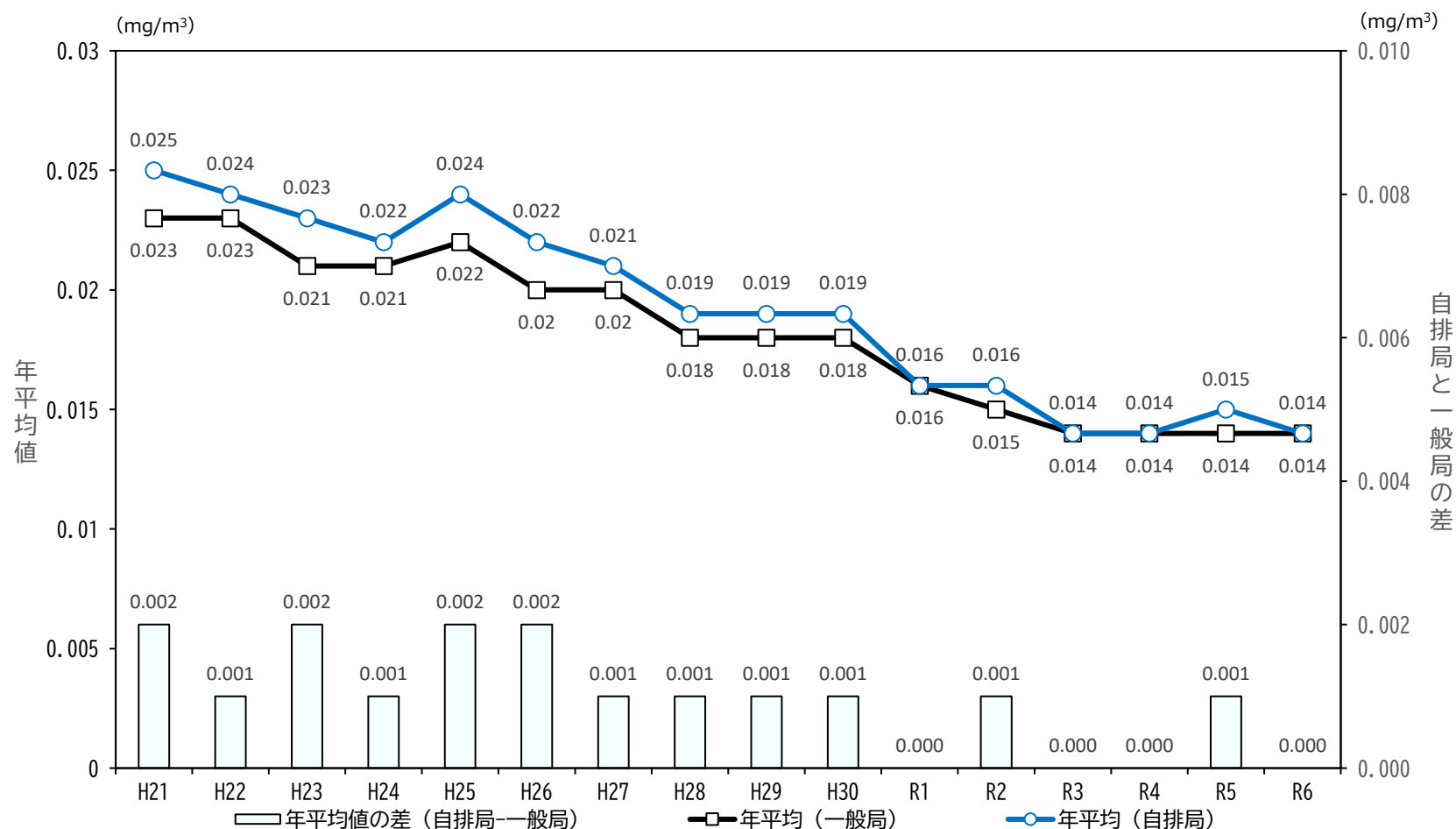
図6.SPM濃度 (年平均値) の経年変化【大阪府全域】
