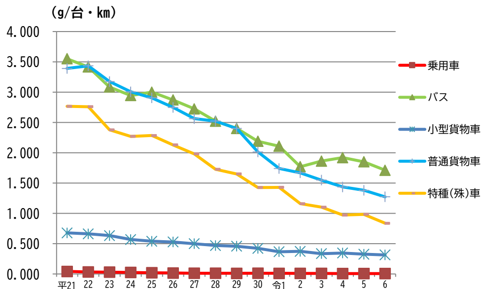
図4. 旅行速度40km/hにおける車種別排出係数 (乗用系、小型貨物系、大型貨物系の主な車種)
