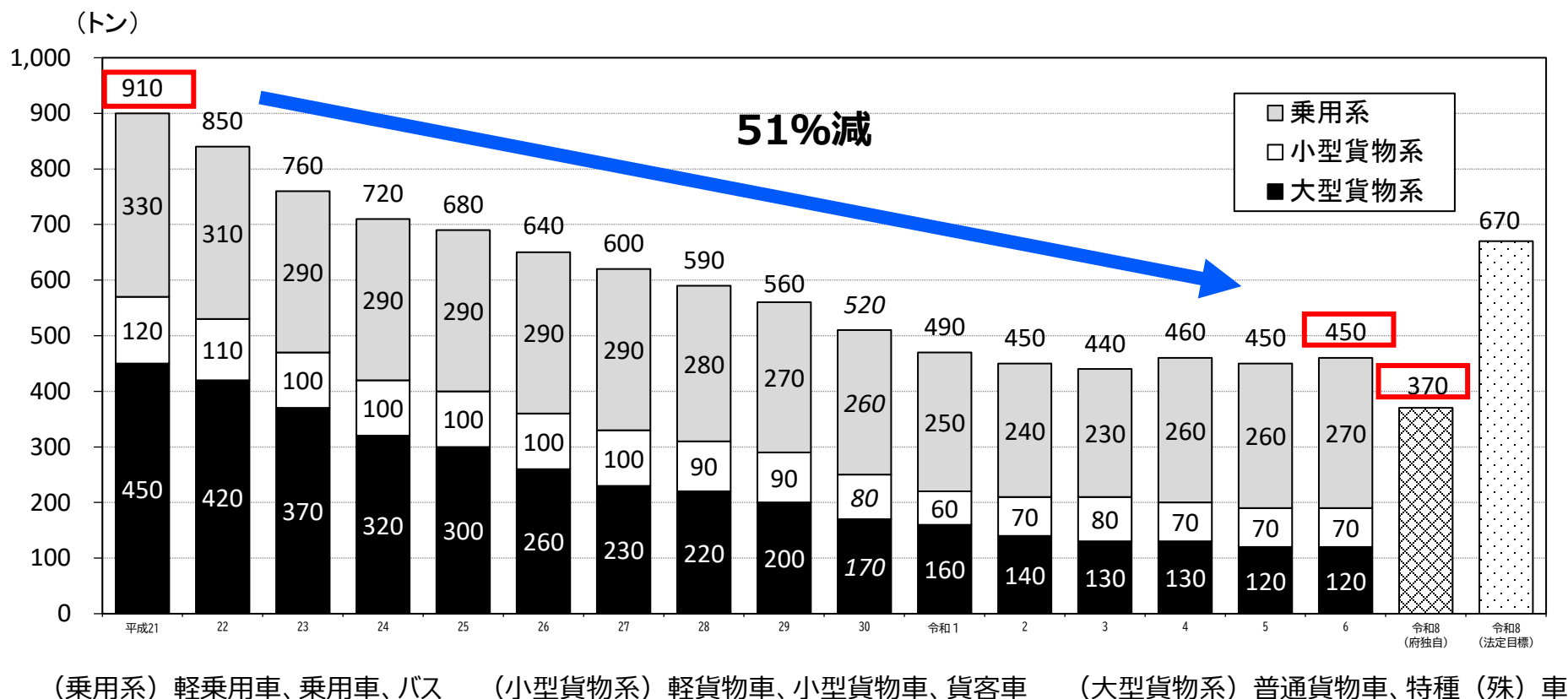
図2. 自動車からのPM排出量の推移 (対策地域)
