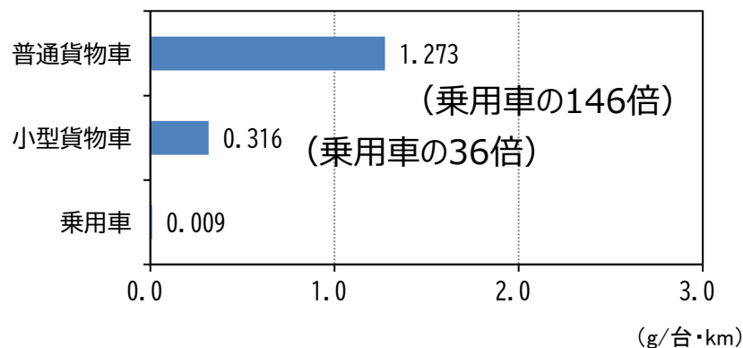
図5. 1 台の車が1km走行時に排出する NOx量（令和6年度）
