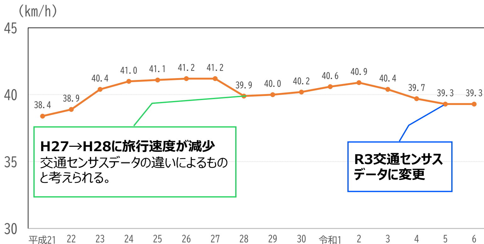
図9. 平均旅行速度（対策地域、全幹線道路）の推移
