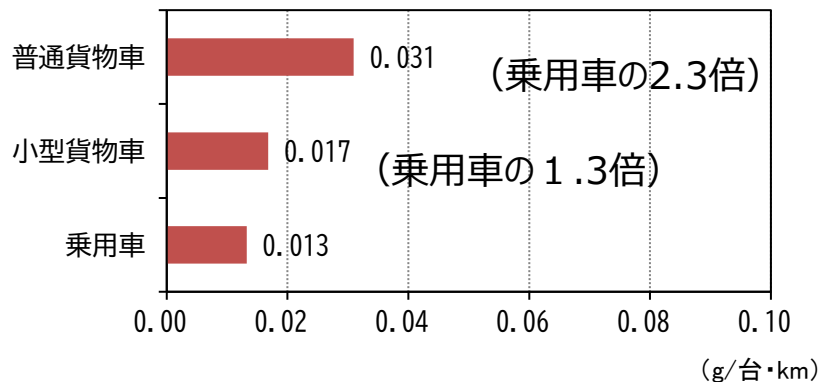
図7. 1台の車が1km走行時に排出する PM量（令和6年度）
