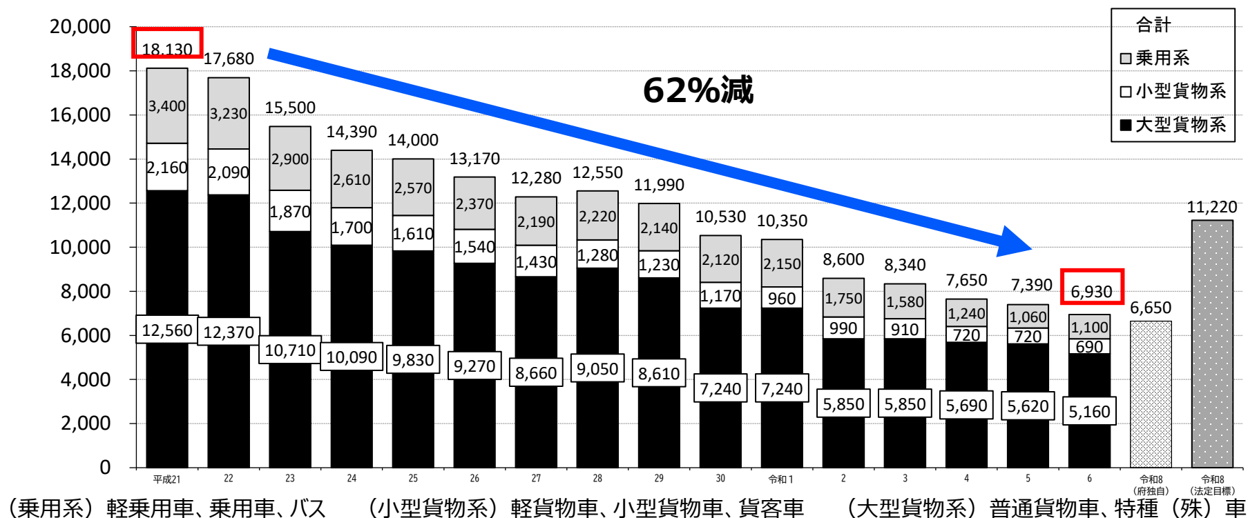
図1. 自動車からのNOx排出量の推移 (対策地域)
