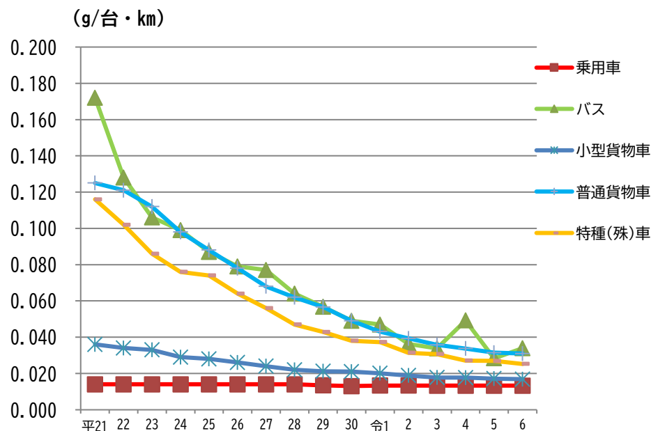
図6. 旅行速度40km/hにおける車種別排出係数 (乗用系、小型貨物系、大型貨物系の主な車種)
