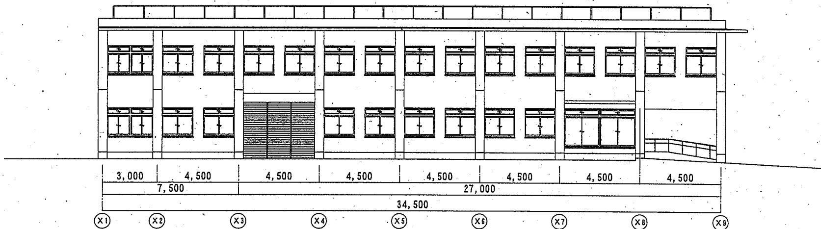
南立面图
