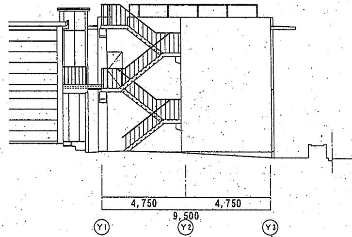
西立面图
