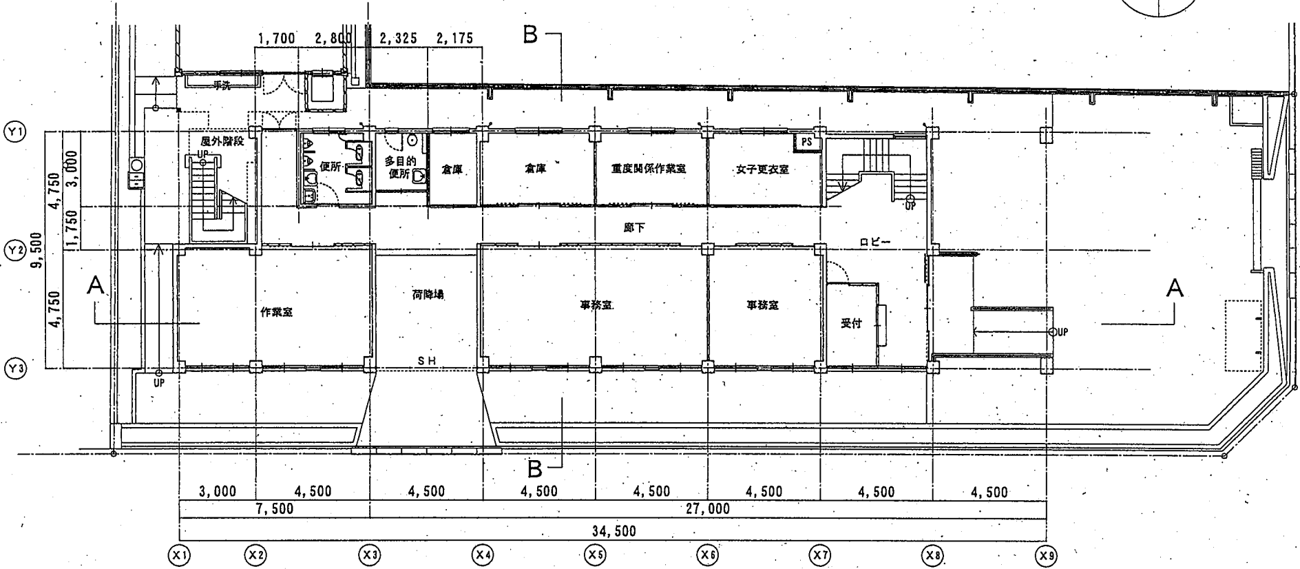
1 階平面図
