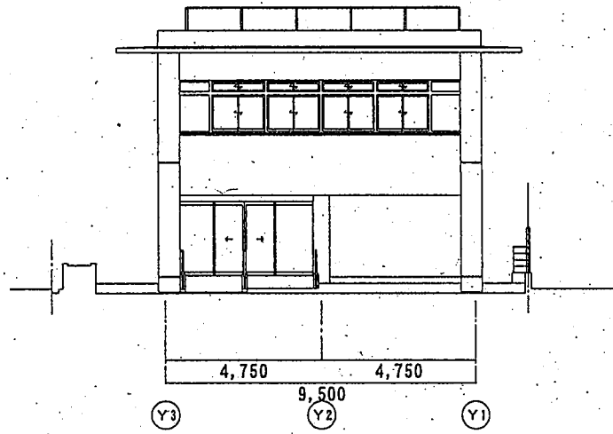
東立面图
