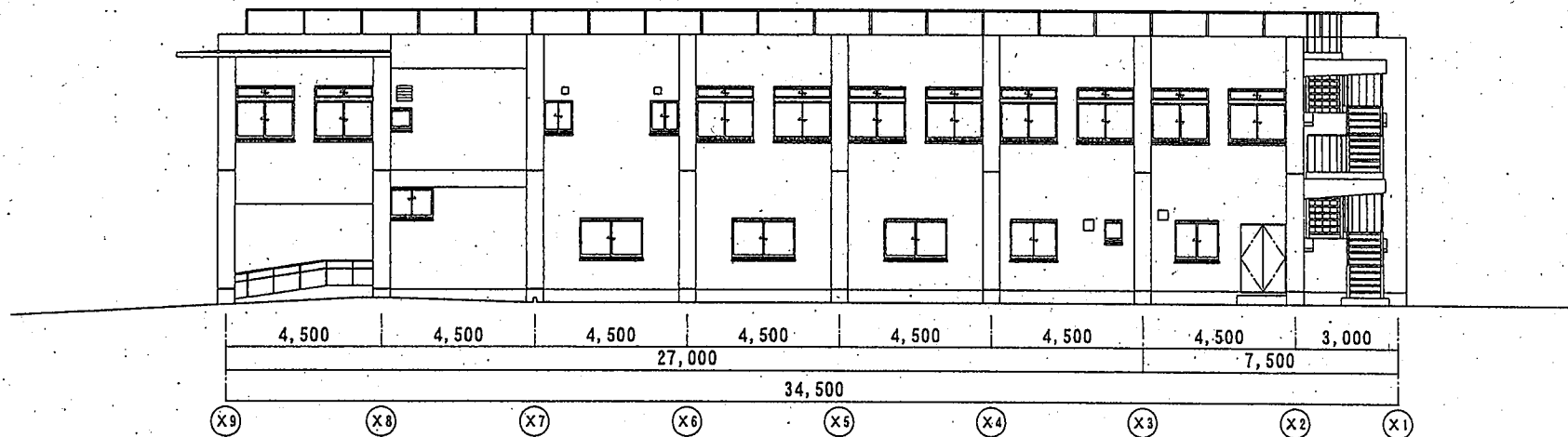
北立面图
