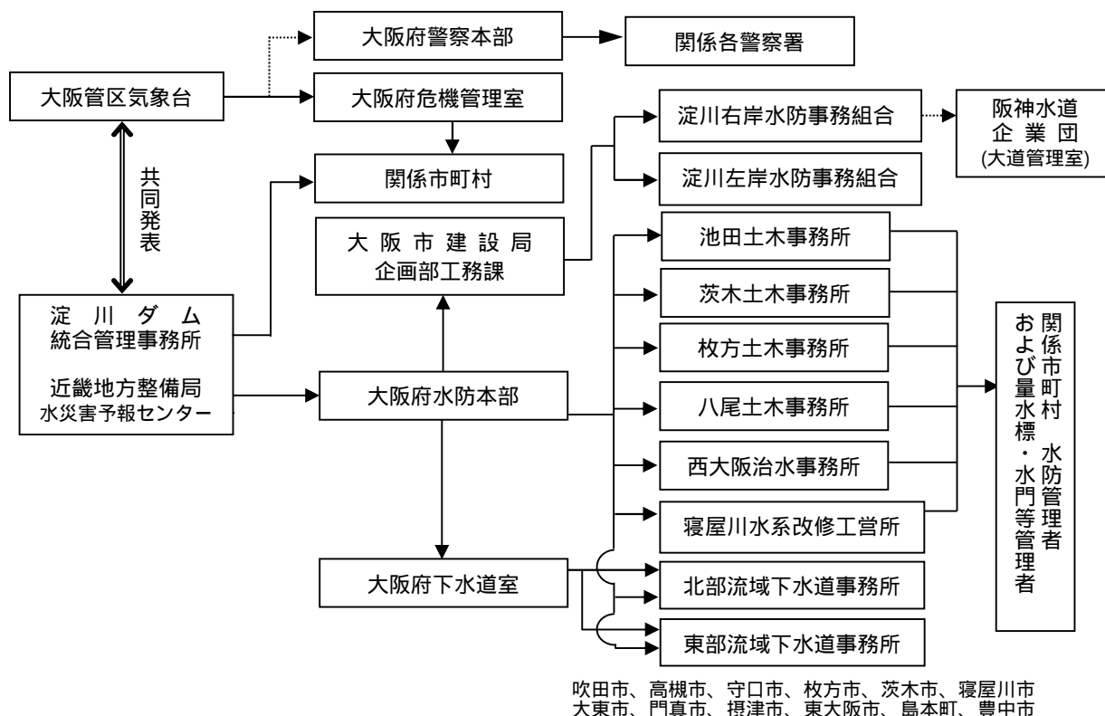
淀川洪水予報通信連絡系統図
