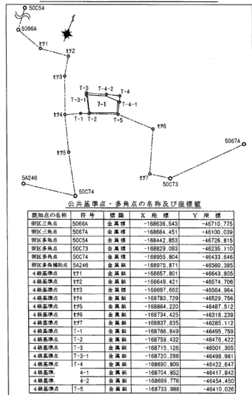
公共基準点・多角点網図 S=1:5000 (2/3)
