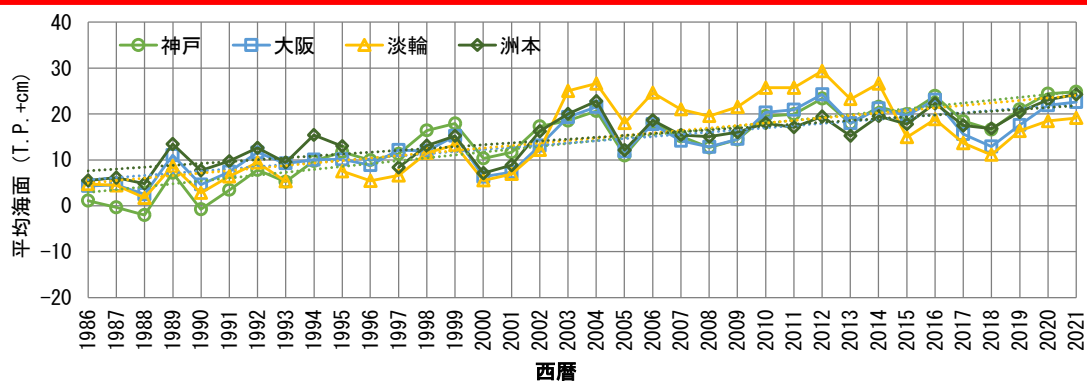
図 1.1.3 平均海面の水位の推移
