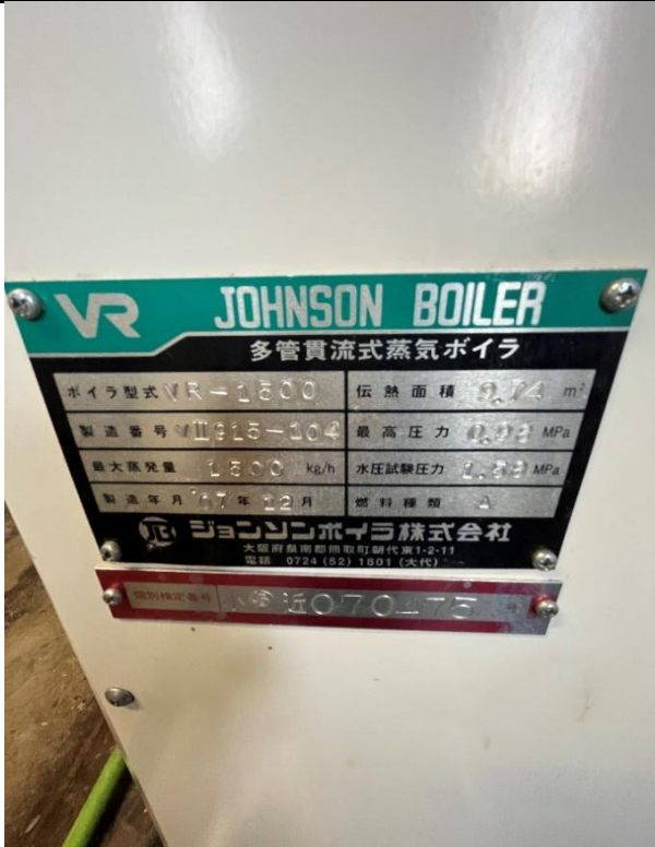
銘板の写真
