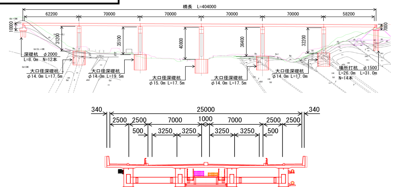
標準断面図
