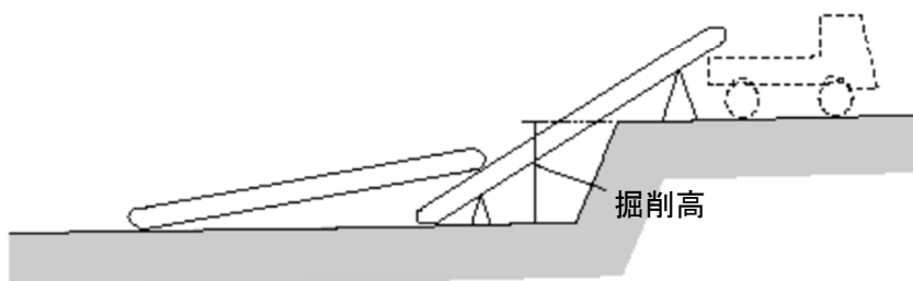
【 調査掘削時のベルトコンベヤ設置例 】
