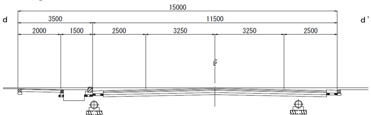
区画道路②
