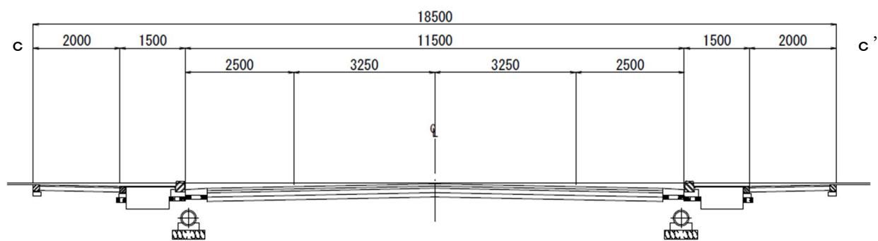
区画道路①
