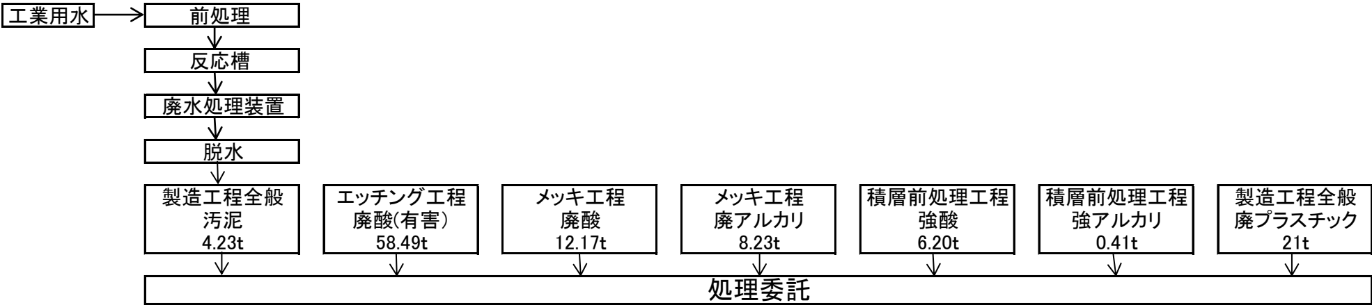
(産業廃棄物発生工程フロー)
