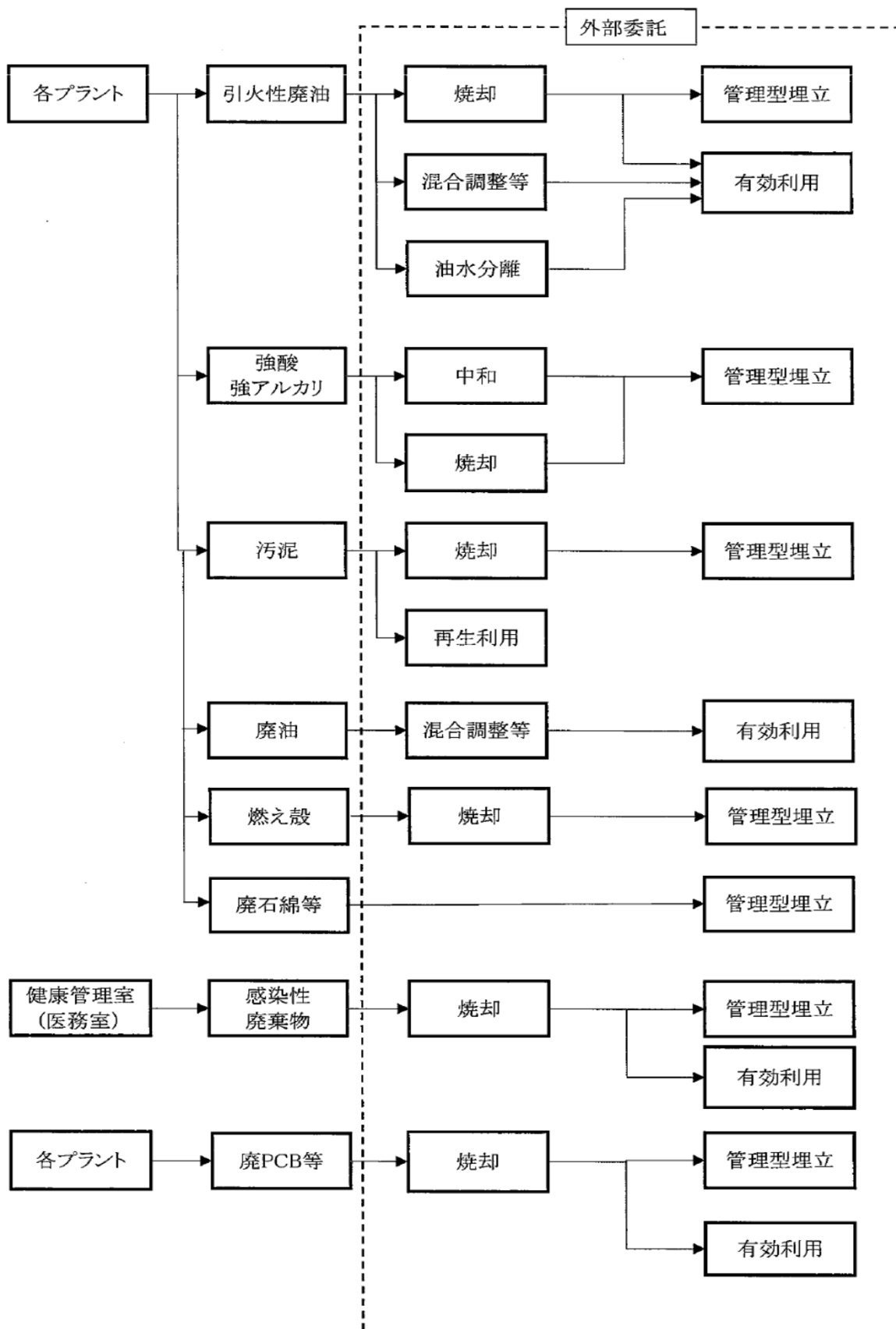
特別管理産業廃棄物処理フロー図
