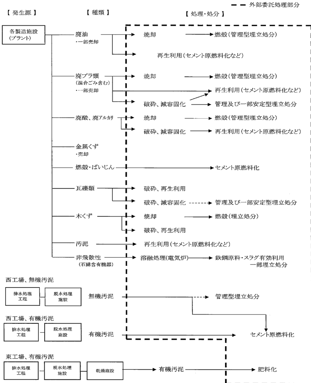
◎ 産業廃棄物処理フロー図
