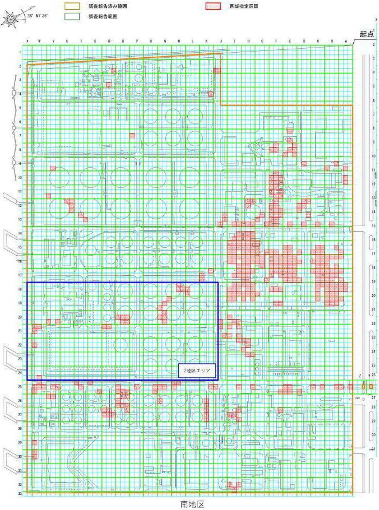
区域指定平面図（敷地全体図）
