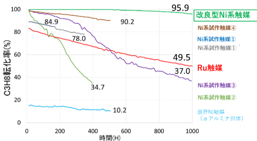
高性能水素製造用水蒸気改質触媒の連続評価結果およびメタン化触媒の温度依存性
