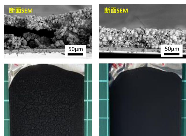
水系正極(NMC811)の外観
