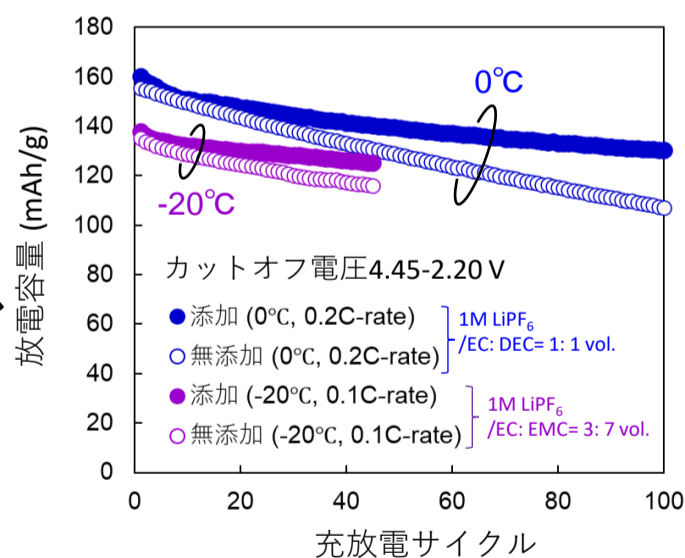
NCA vs. SiOセルのサイクル特性
