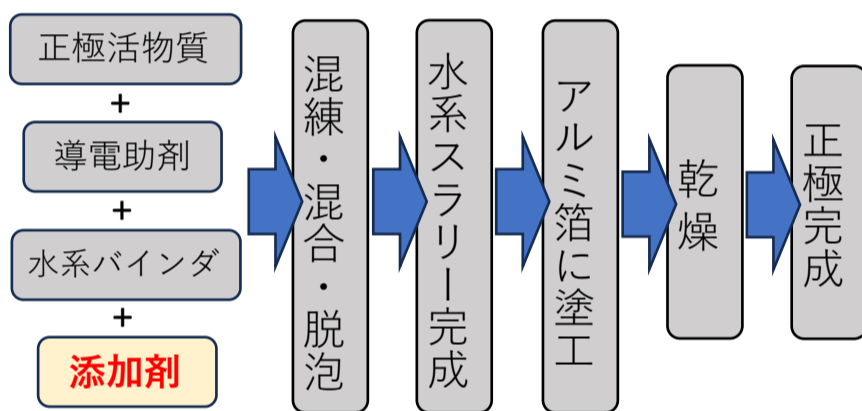
添加剤の適用プロセス
