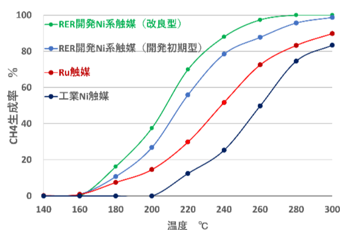
高性能水素製造用水蒸気改質触媒の連続評価結果およびメタン化触媒の温度依存性
