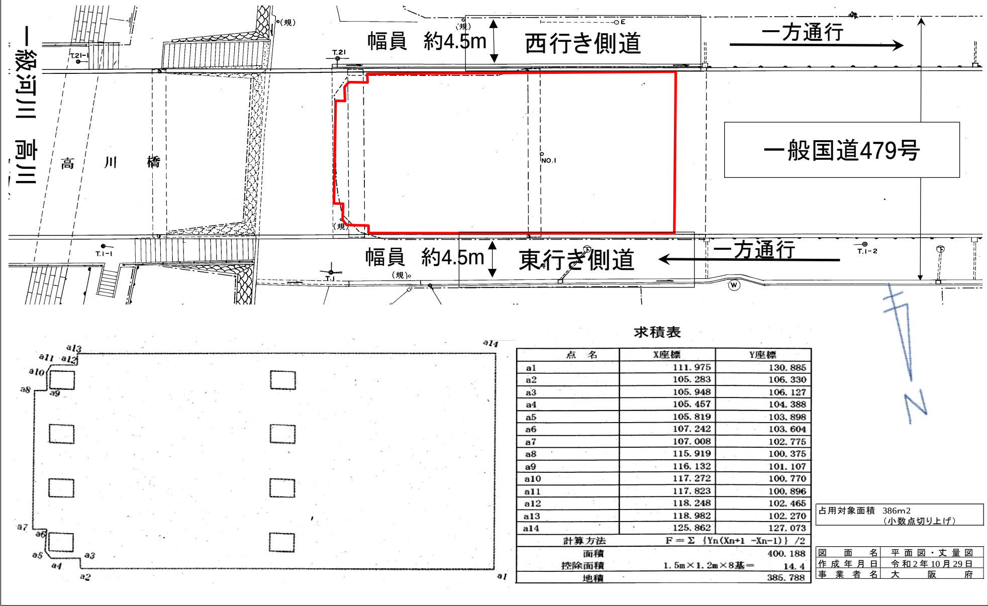
(2) 平面図・丈量図 (物件番号：第1号)
