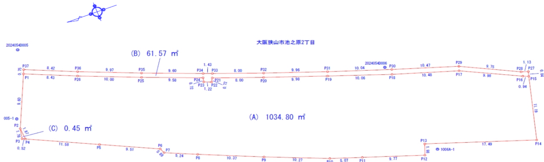
貸付範囲 (A) 丈量図
