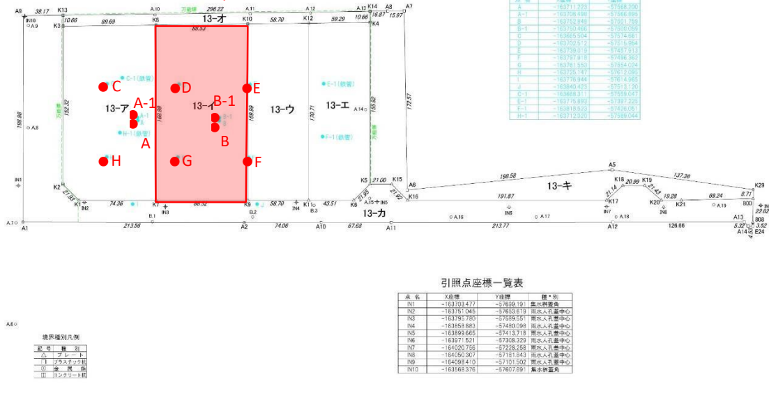
ガス抜孔位置・座標一覧表
