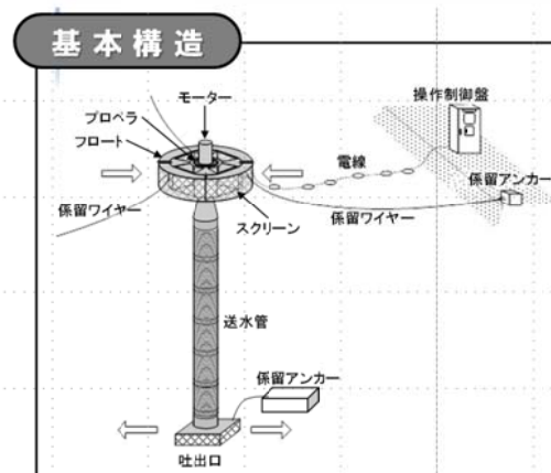
写真 4.2-1 フロベラ式湖水循環装置 (出典：パンフレット)
