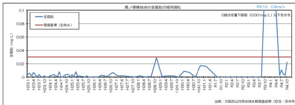
図 4-7 全亜鉛の経年変化（桑原橋）
