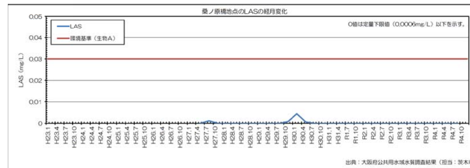
図 4-9 LASの経年変化（桑原橋）
