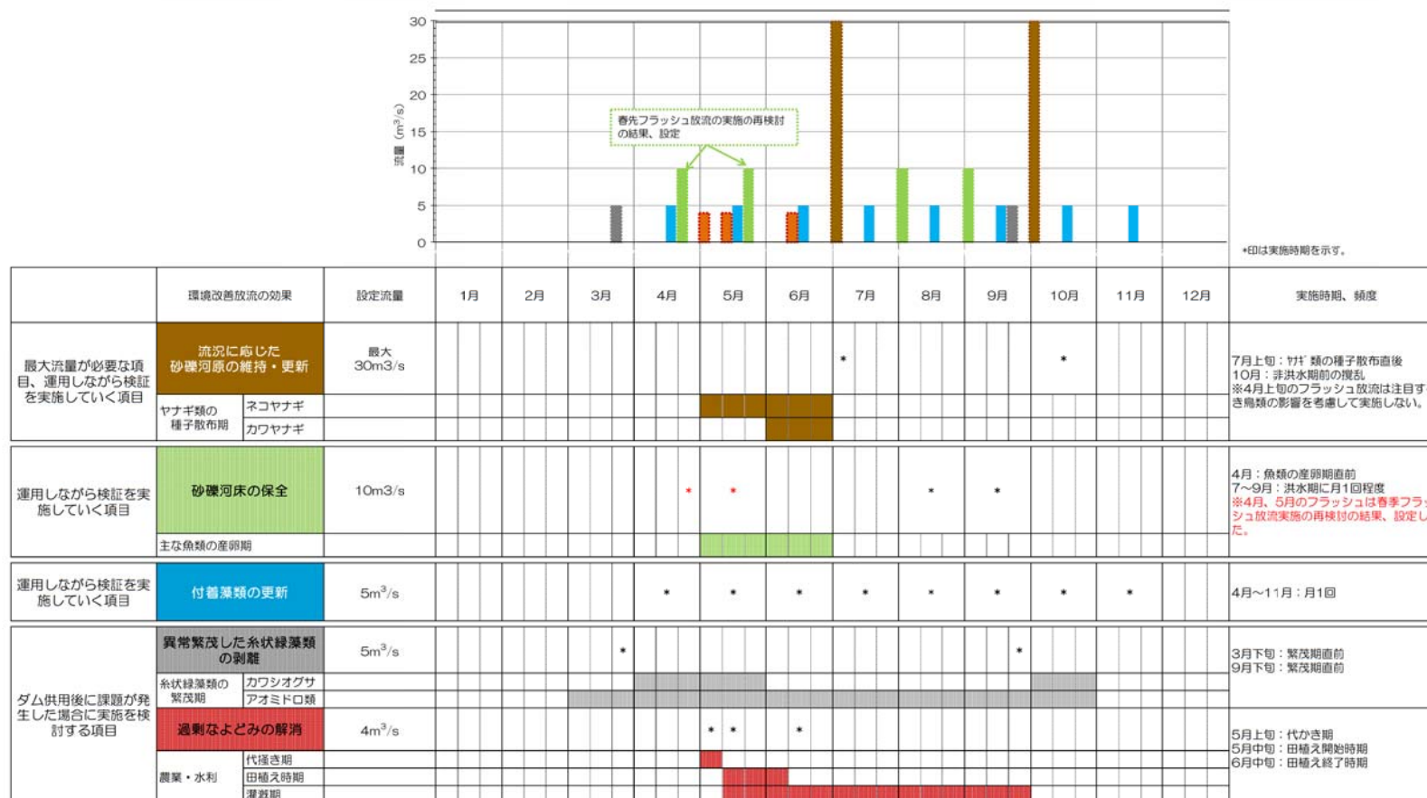
図 4-10 フラッシュ放流年間放流パターン（R4.3 版）
