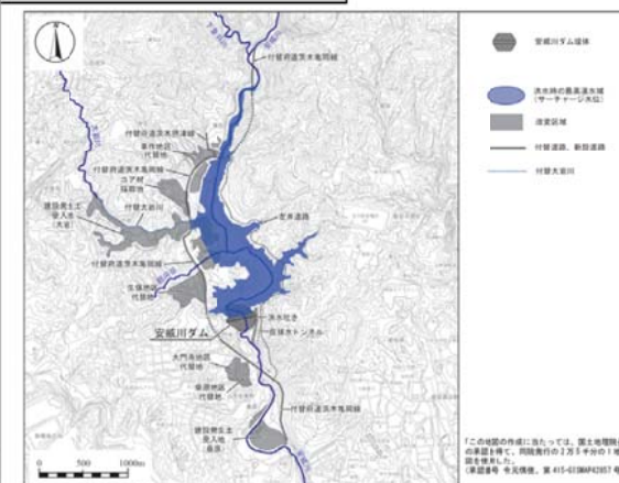
図 4-2 サーチャージ水位のイメージ
