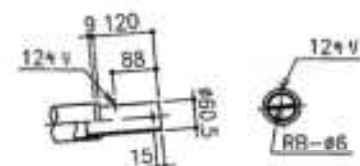
アダプター詳細図 S=1:10
