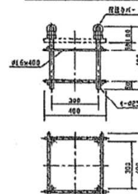
アソカーボルト詳細図 S=1/10
