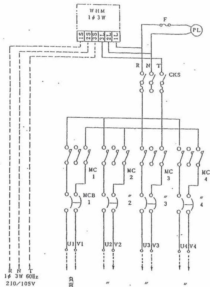
結 線 図
