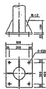
アソカーボルト詳細図 S=1/10
