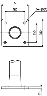
柱脚部詳細 S=1/10
