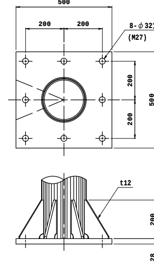
柱脚部詳細 S=1:10
