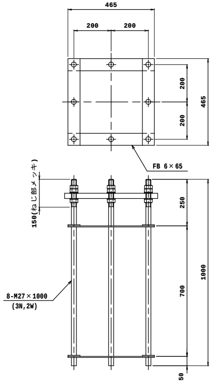
アンカーフレーム S=1:10
