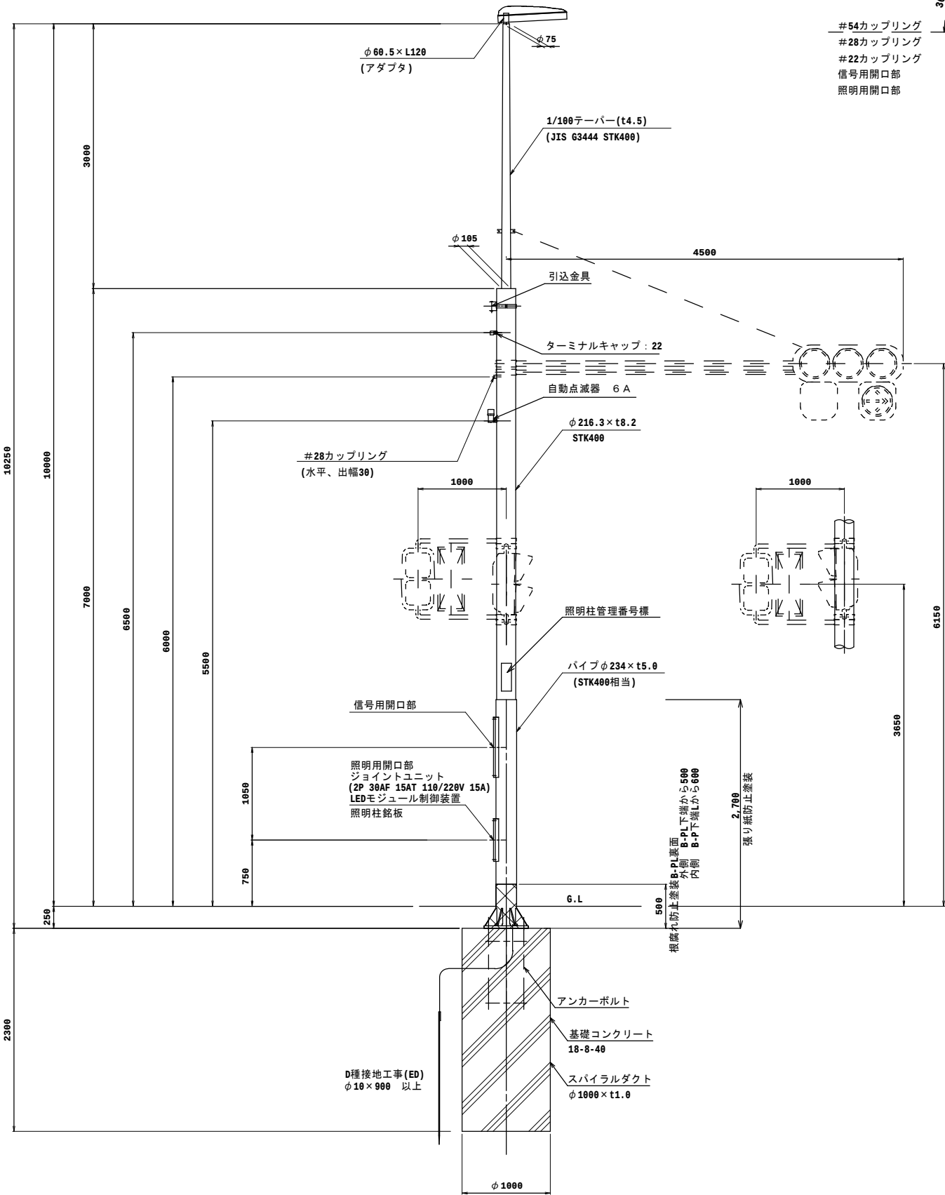
姿図 S=1:30
