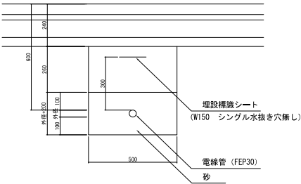
埋設配管要領図 S=1/10 (一般部)
