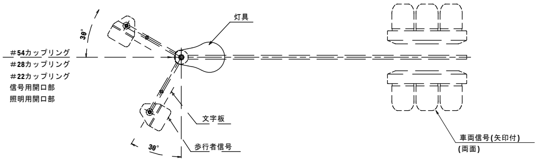
平面図
