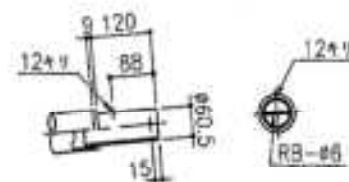
アダプター詳細図 S=1:10
