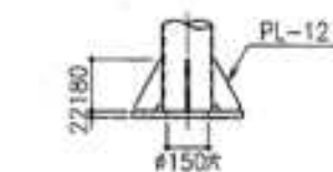
ベースプレート詳細図 S=1:20
