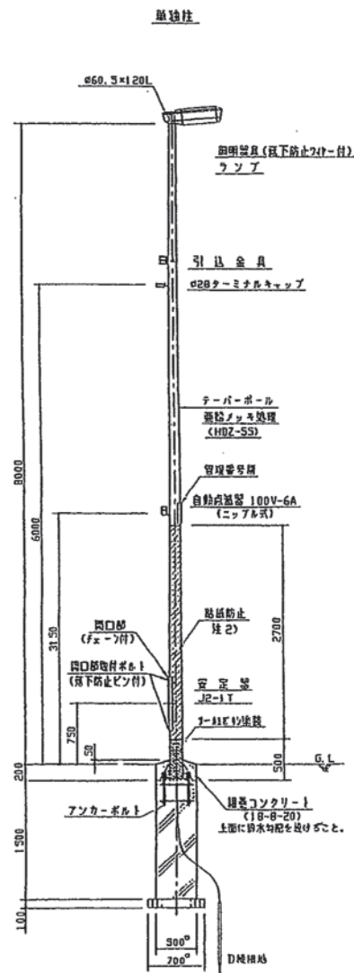
照明柱詳細図 S=1/30
