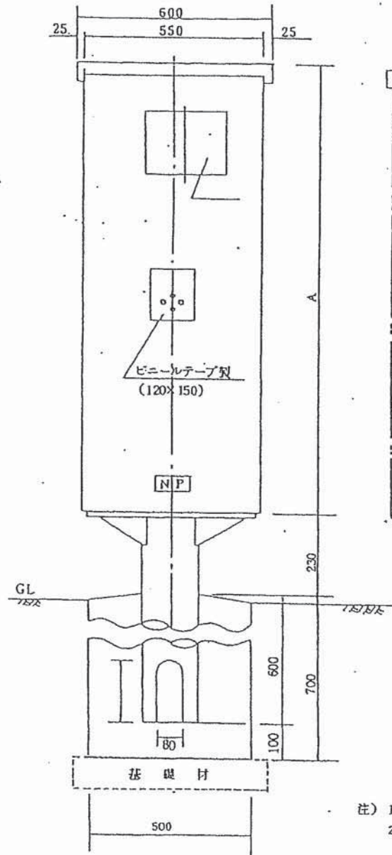
正面図
