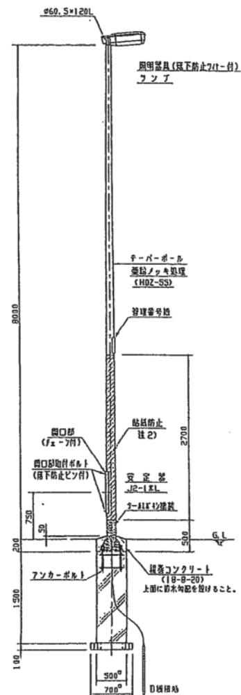
連続柱
