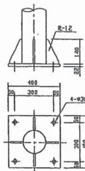
アソカーボルト詳細図 S=1/10
