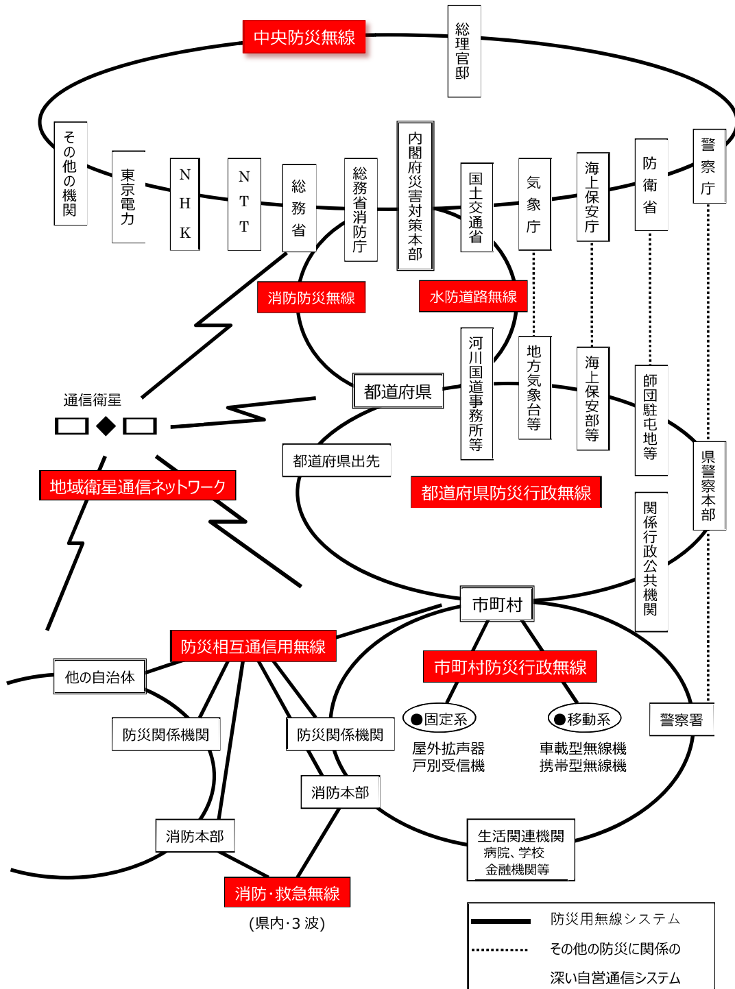
防災用通信システムの全体構成図
