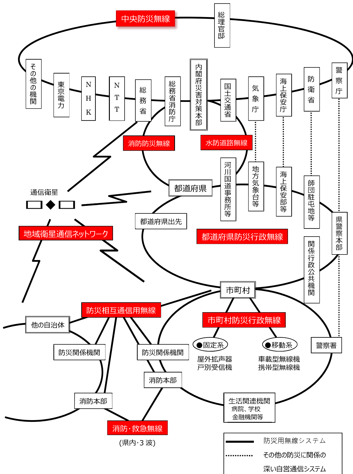
防災用通信システムの全体構成図
