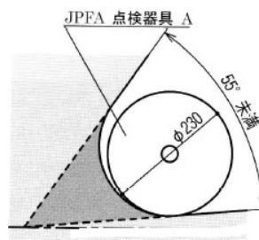
図16 開口部の隅角部を埋めた対策 点検器具がV字2辺に接しない事が必要
