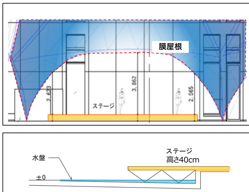
(ステージ立面図)
