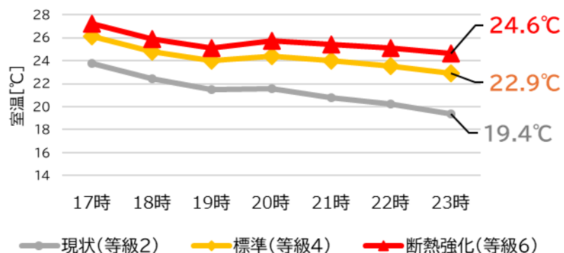
図表 16 「空調を使用しない時期の室温変化（中間期）」の出力例（新築）
