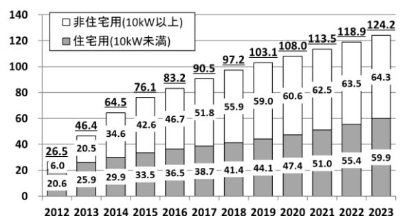
府内における太陽光発電設備導入量の推移
