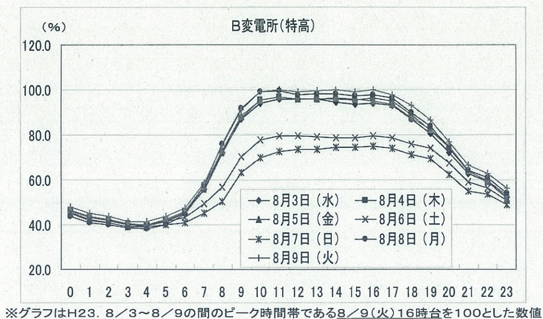
B変電所の負荷曲線（主に商業地）
