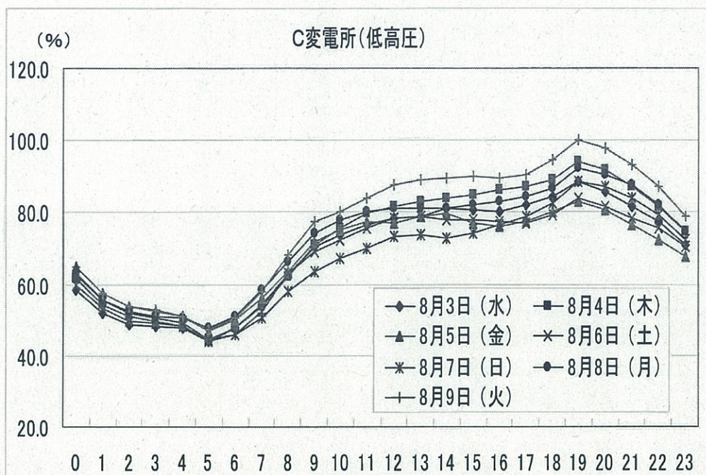
図 30 変電所における夏期の電力需要曲線の事例（2）
