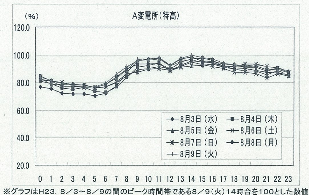
A変電所の負荷曲線（主に工業地）
