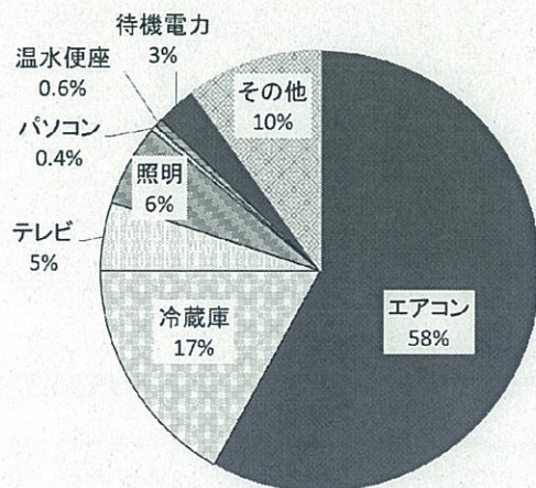
図 31 家庭（在宅世帯）の用途別電力需要（夏期、14 時頃）
