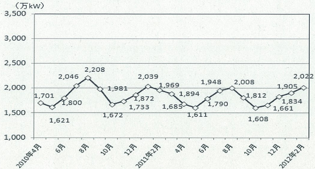
図22 月別の平均電力需要
