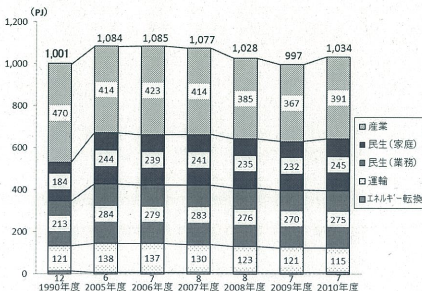
図4 府域の部門別エネルギー消費量 (一次エネルギーベース) の推移
