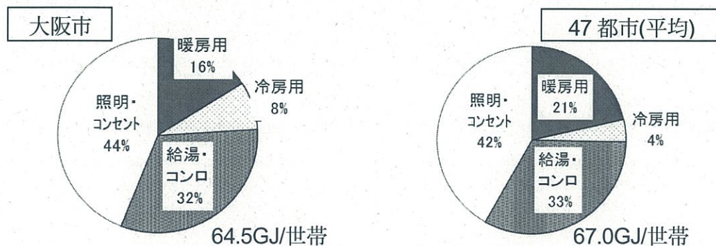
図 12 家庭における用途別エネルギー消費量 (一次エネルギーベース)
