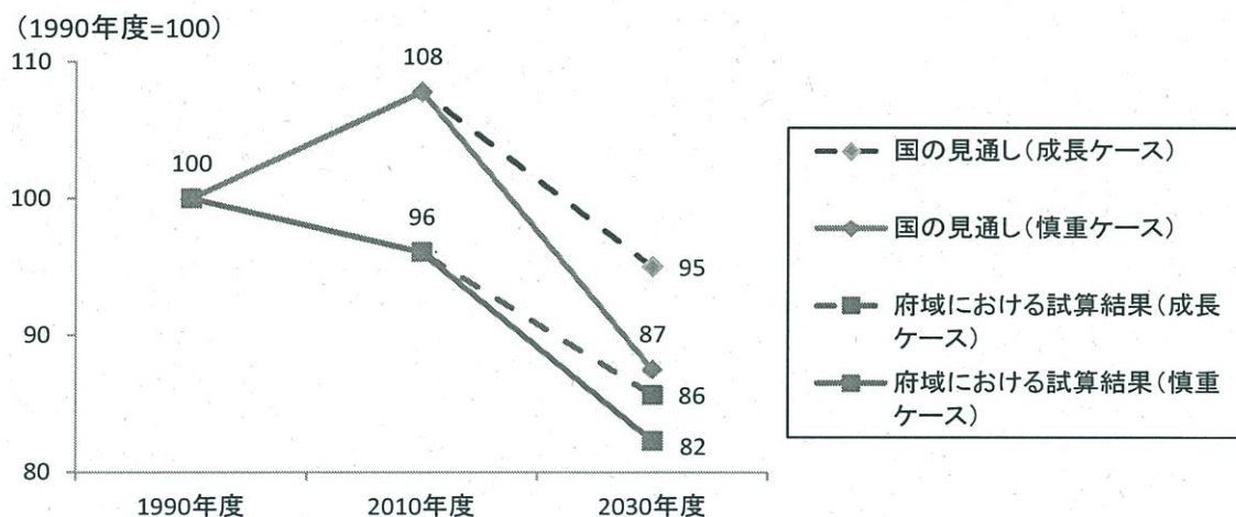
図9 エネルギー消費量に係る府域における試算結果と国の見通しとの比較
