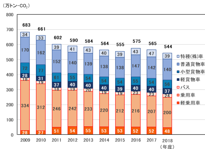
自動車の二酸化炭素排出量の推移 (大阪府域)
