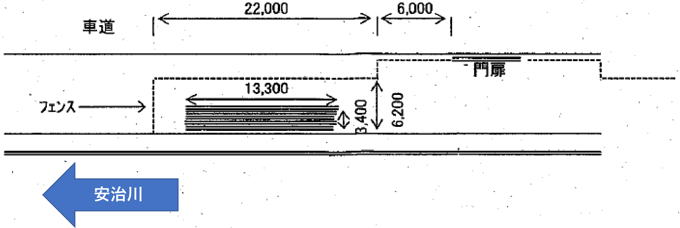
○平面図
