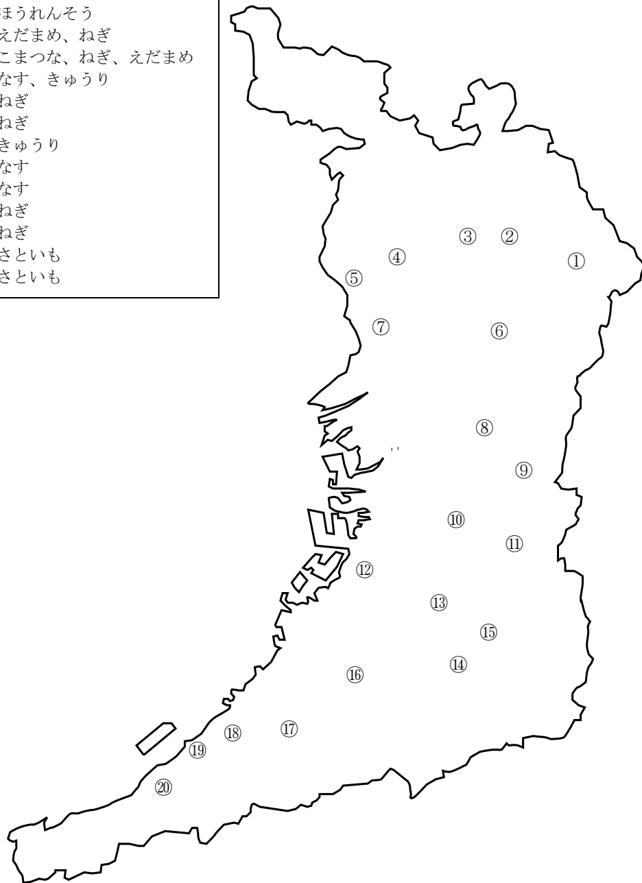
図1-3-1 農作物影響調査地点設置図（平成21年度）
