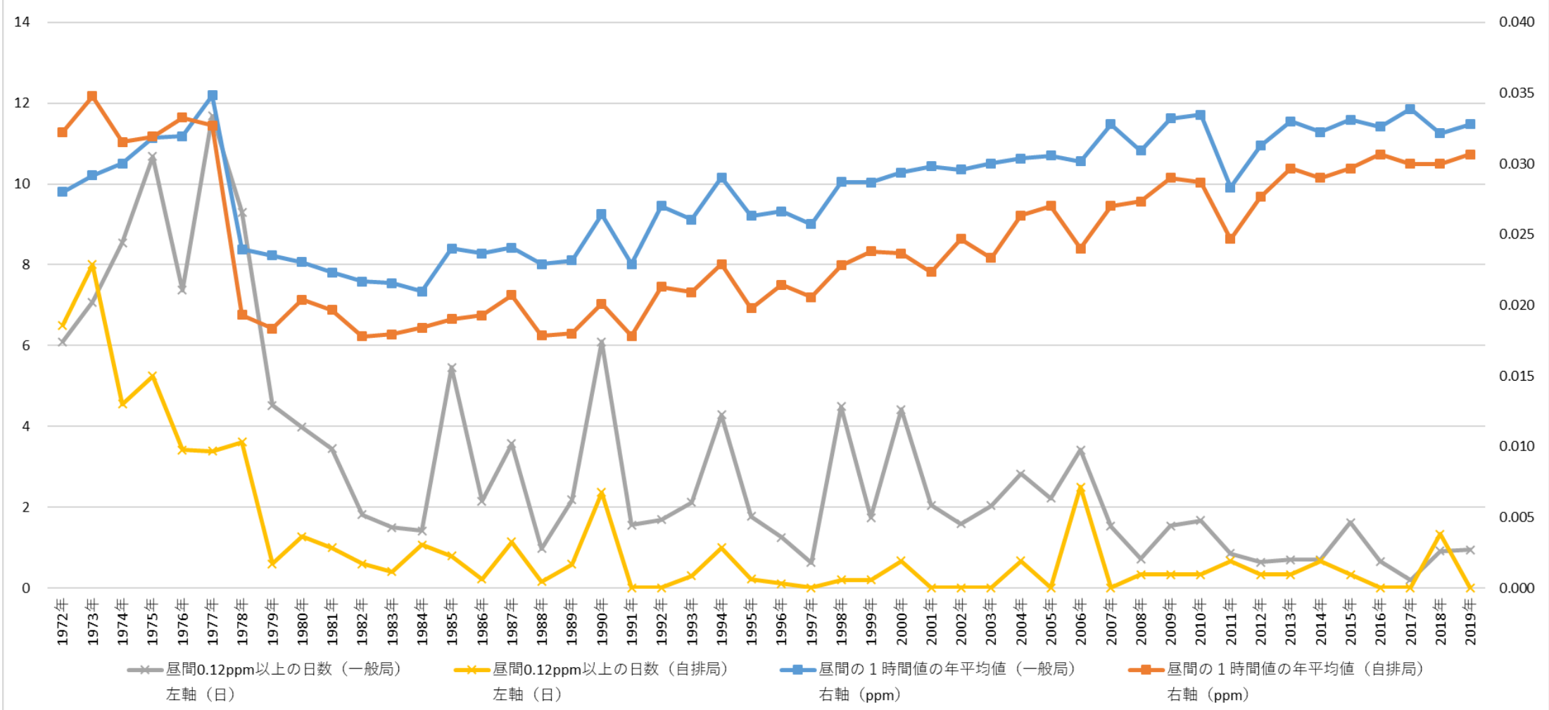
大阪府内におけるオキシダントの推移（1972～2019年）
