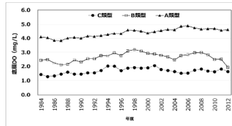
図5 底層DOの年度最小値の経年変化(5年間移動平均)
