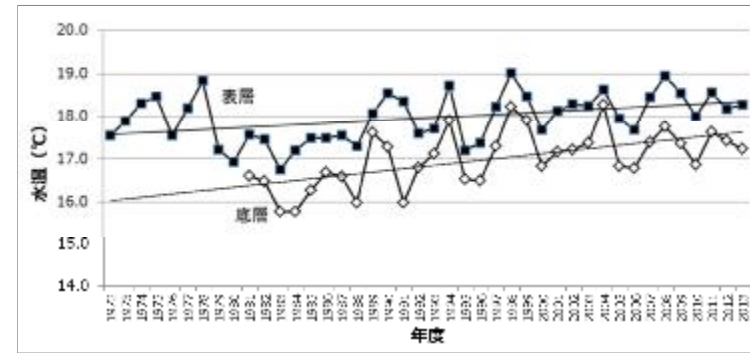
図3 大阪府が測定する環境基準点の水温の推移(年平均値; 湾東部12地点)
