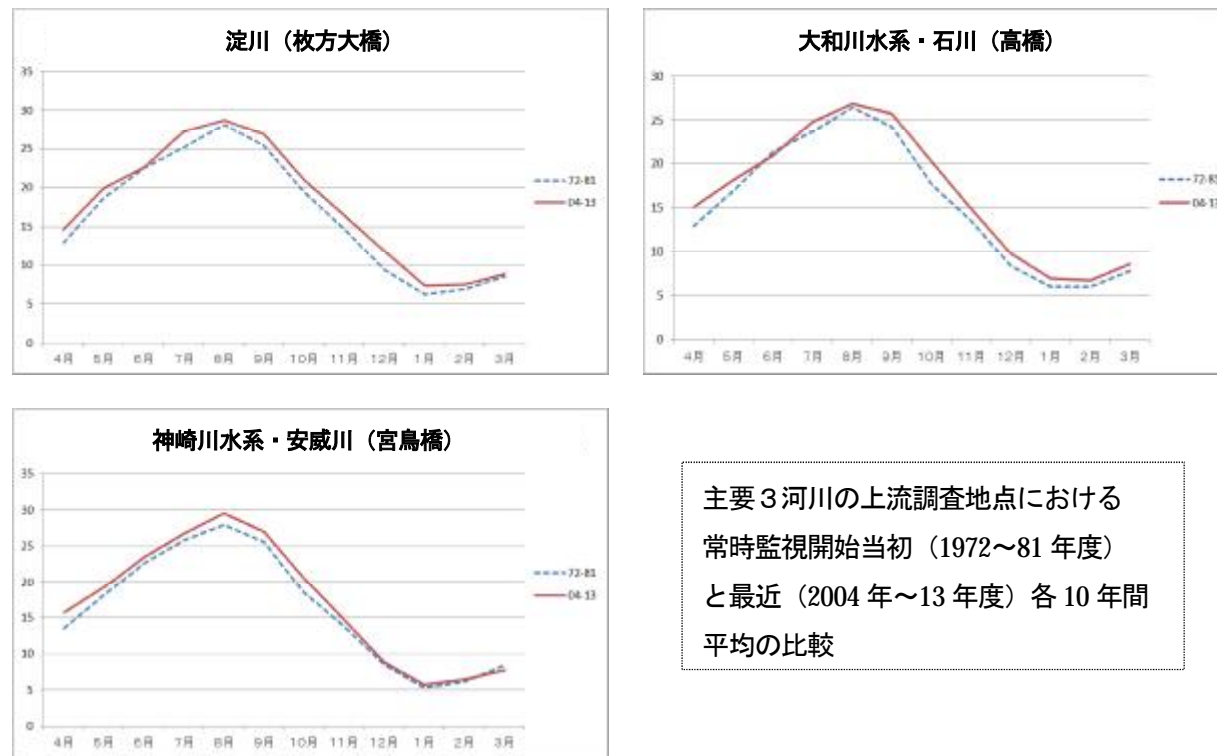
図2 大阪府内主要河川・上流地点における月別水温の経年比較
