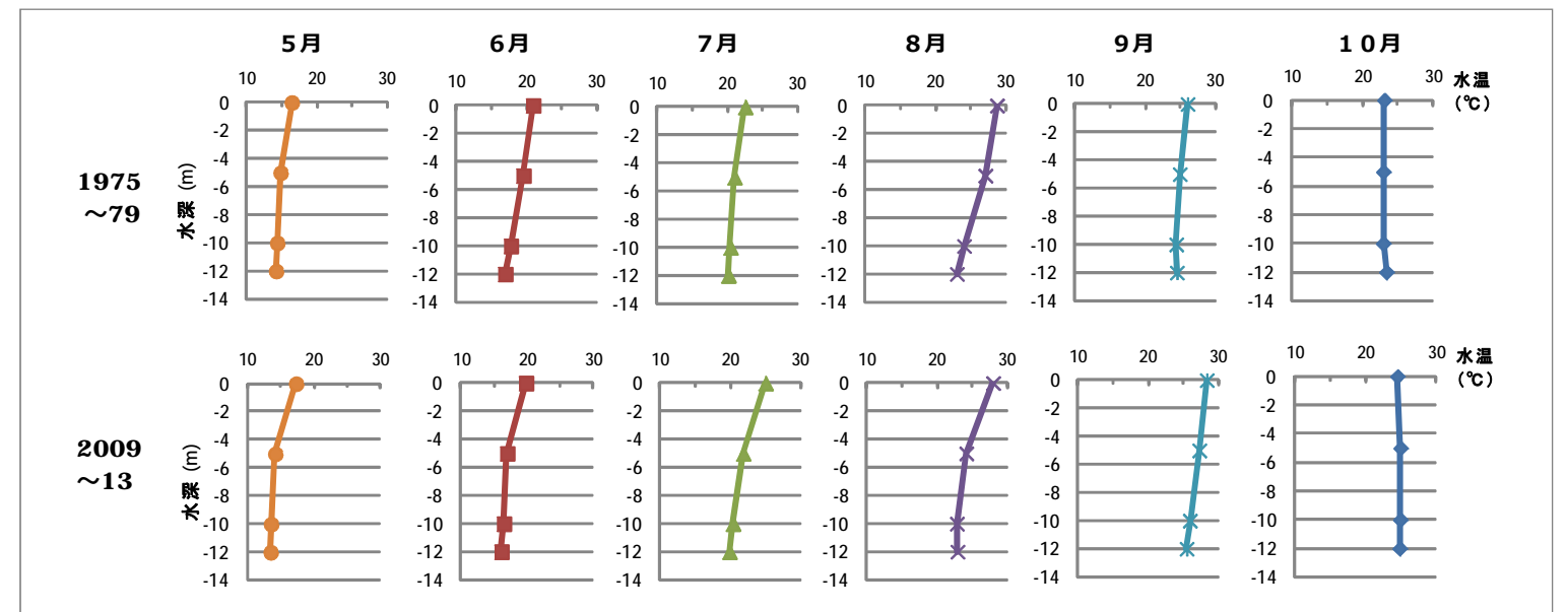
図6 大阪湾・湾奥部における成層化の状況 (湾奥部(st. 18、浅海定線)における月別の水温鉛直プロファイルの1975~79年、2009~13年の各5年間の平均経年変化)
