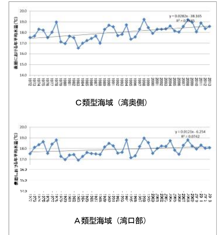
図4 表層における年平均水温の推移
