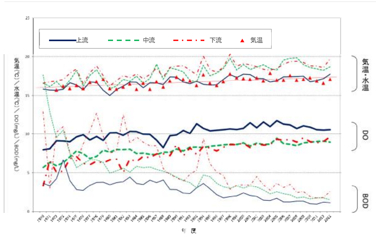
図1 大阪府内主要河川における気温+水温とDO・BODの推移 (淀川、大和川、神崎川の各上・中・下流の平均値、大阪管区気象台の気温)
