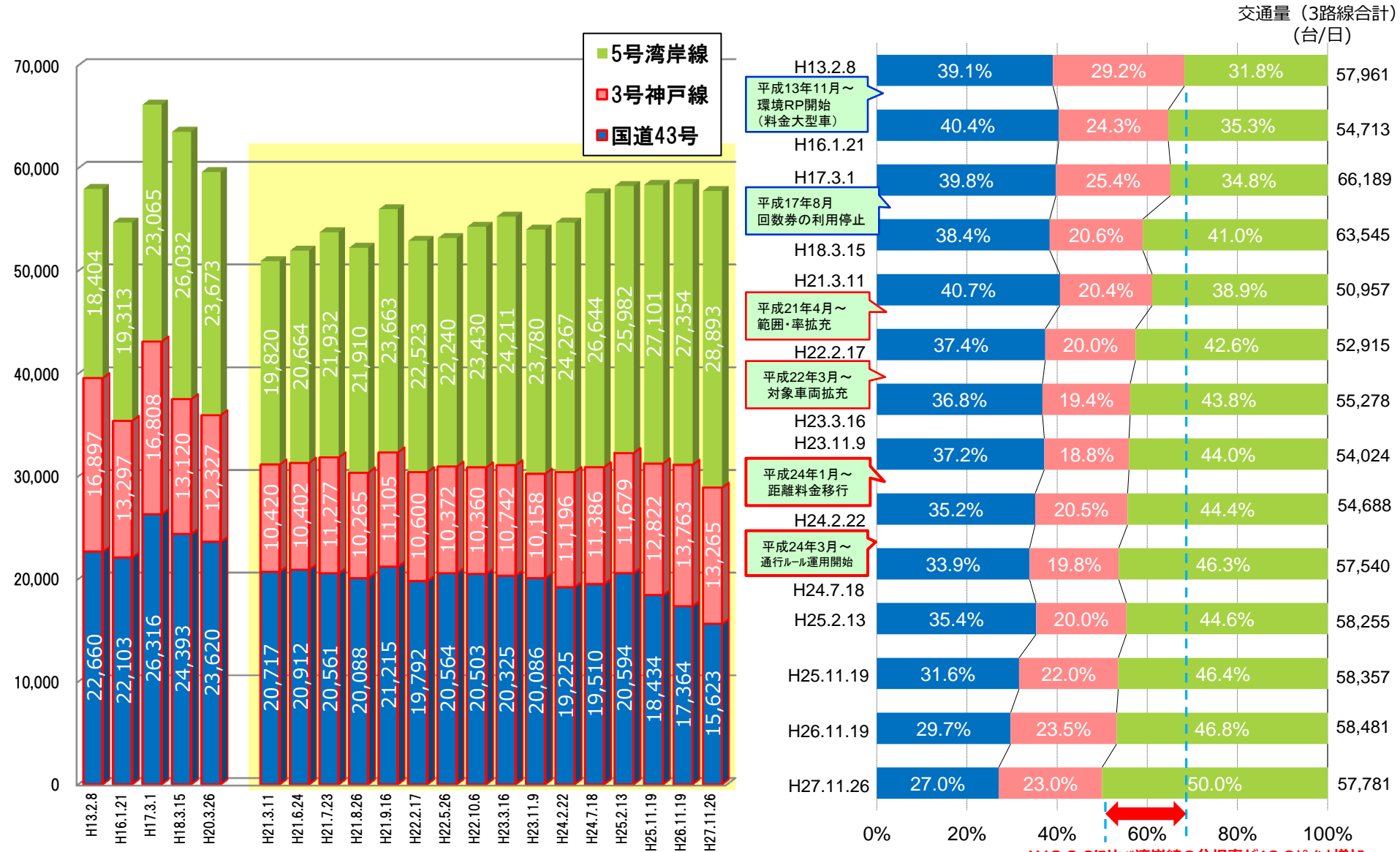
断面交通量 (台/日)
