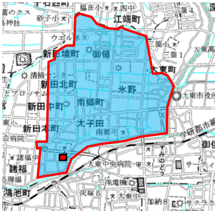
東諸福調節池 集水区域図
