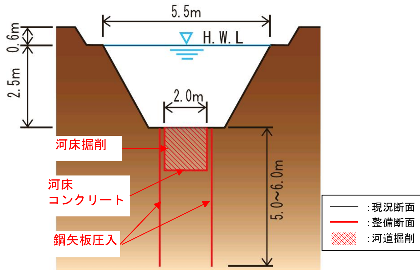
整備断面例 (1.6km地点)
