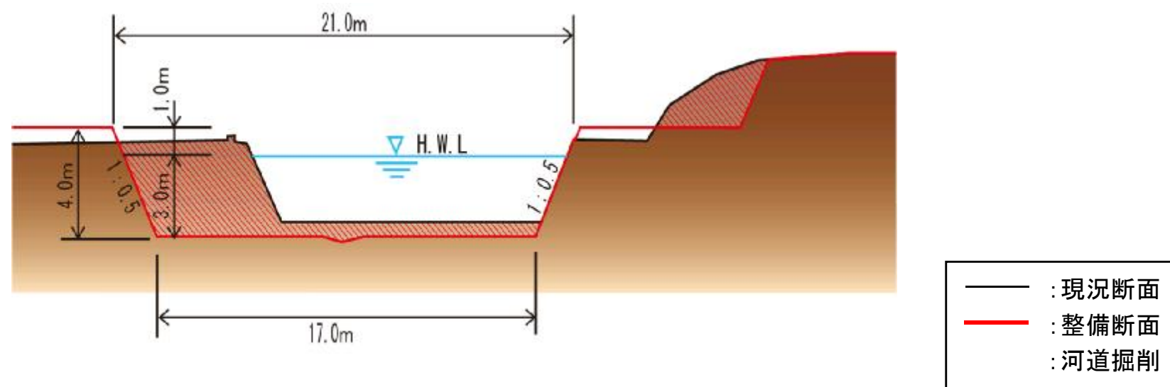
整備断面例 (10.0km地点)
