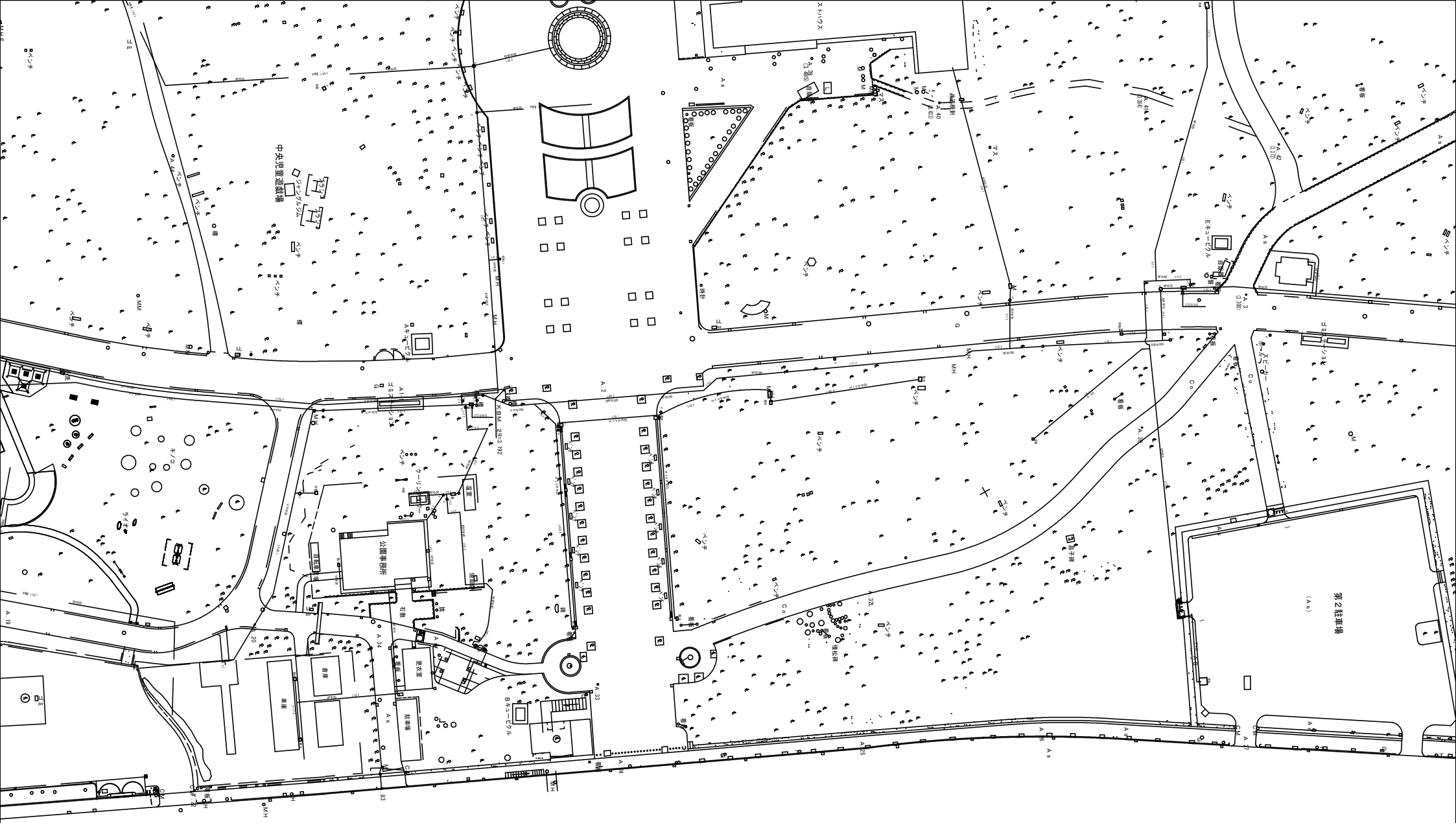
現地説明会配布資料 地下埋設図1/4 浜寺公園 給水・井水施設平面図
